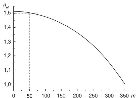
Рис. 2. Зависимость от индекса мод подложки. Расчет по ф. (8) для h_s = 100 мкм
