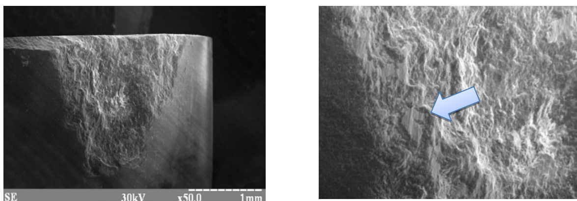
Рис. 6. Зношення ріжучої пластини по задній поверхні
