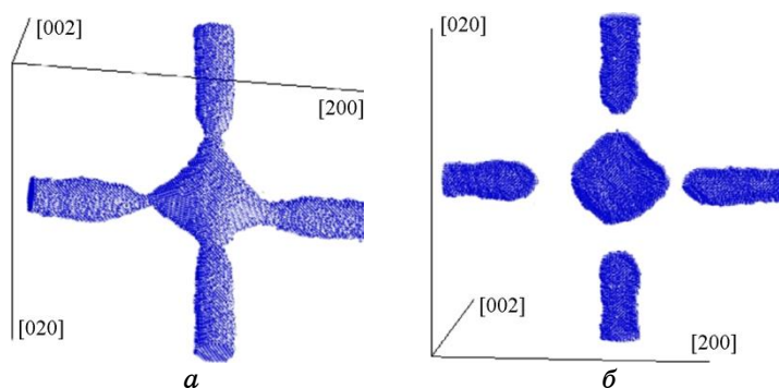
Рис. 4. Эволюция контакта при отжиге нанопроволок с радиусами R_1 = R_2 = 12a , ориентациями [200] и [020], углом взаимной ориентации 90^\circ в моменты времени: (а) 2,5 \cdot 10^5 МКШ и (б) 4,1 \cdot 10^5 МКШ.
