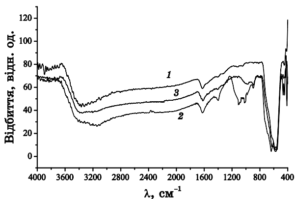
Рис. 1. ІЧ-Фур'є-спектри вихідного (немодифікованого) магнетиту \text{Fe}_3\text{O}_4 ( а ), наноккомпозитів \text{Fe}_3\text{O}_4/\text{SiO}_2 (ХМ) ( б ) та \text{Fe}_3\text{O}_4/\text{SiO}_2 (АМ) ( в ).
