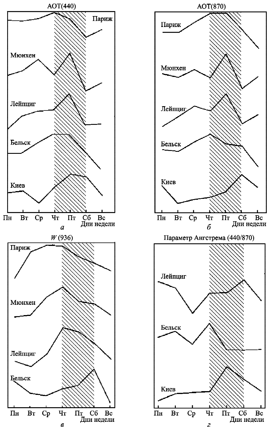
Рис. 6. Сравнительный анализ недельной цикличности АОТ(440) (а), АОТ(870) (б), W(936) (в) и параметр Ангрстрема (440/870) (г) для различных населенных пунктов
