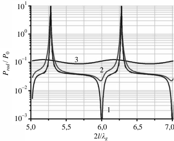
Рис. 6. Радиационные потери мощности ЗДДР на шелевом ЭС с поршнем в волноводе
