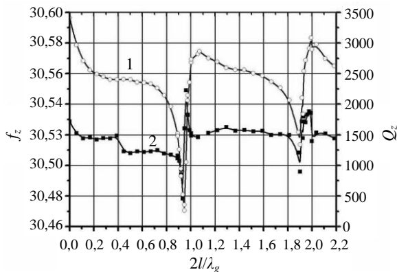
Рис. 8. Добротность (кривая 1) и относительный сдвиг частоты (кривая 2) ЗДДР, связанного через отверстие в диафрагме с короткозамкнутым волноводом
