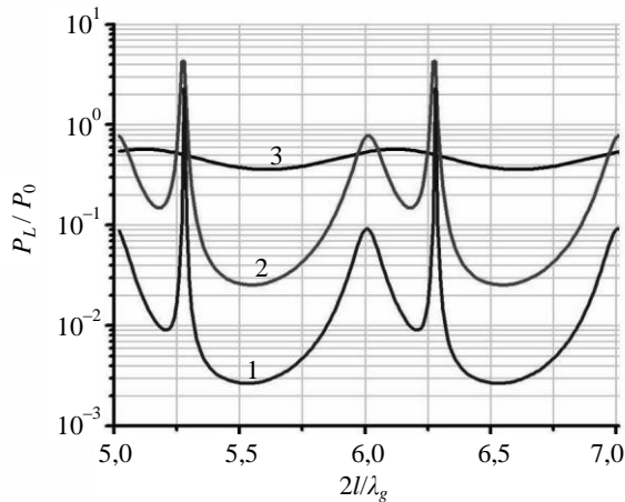
Рис. 7. Потери мощности в активном сопротивлении поршня в волноводе, связанном с ЗДР шелевым ЭС
