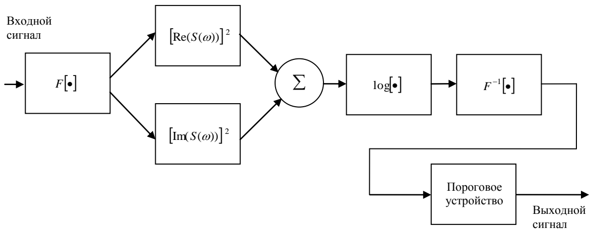
Рис. 5. Структура алгоритма гомоморфной обработки сигналов георадара
