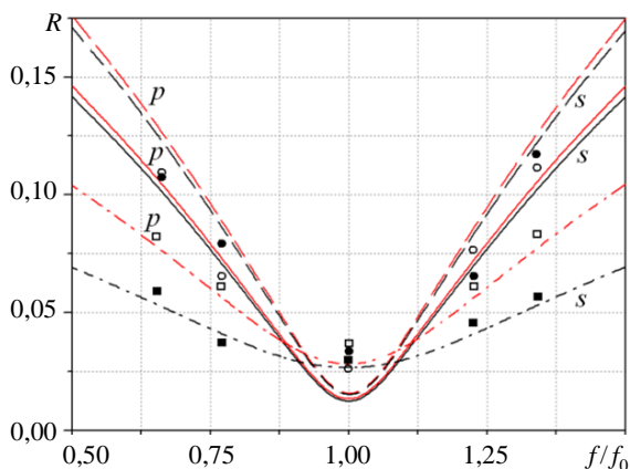
Рис. 3. Частотные зависимости коэффициентов отражения от полубесконечных структур при «изотропном согласовании»: сплошные кривые – лавсан–тефлон при выступающем тефлоне (о, ● – соответственно экспериментальные значения R_p и R_s ); пунктирные кривые – лавсан–тефлон при выступающем лавсане и штрих-пунктирные – полистирол–воздух (□ – R_p , ■ – R_s )
