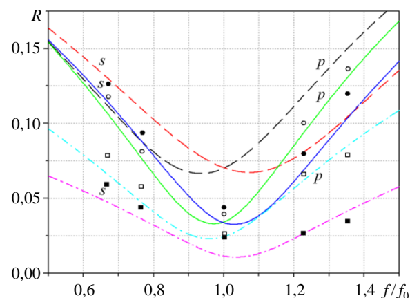
Рис. 5. Частотные зависимости коэффициентов отражения от полубесконечных структур при «анизотропном согласовании»: сплошные кривые – лавсан–тефлон при выступающем тефлоне ( \circ , \bullet – соответственно экспериментальные значения R_p и R_s ); пунктирные кривые – лавсан–тефлон при выступающем лавсане ( \square – R_p , \blacksquare – R_s ) и штрих-пунктирные – полистирол–воздух
