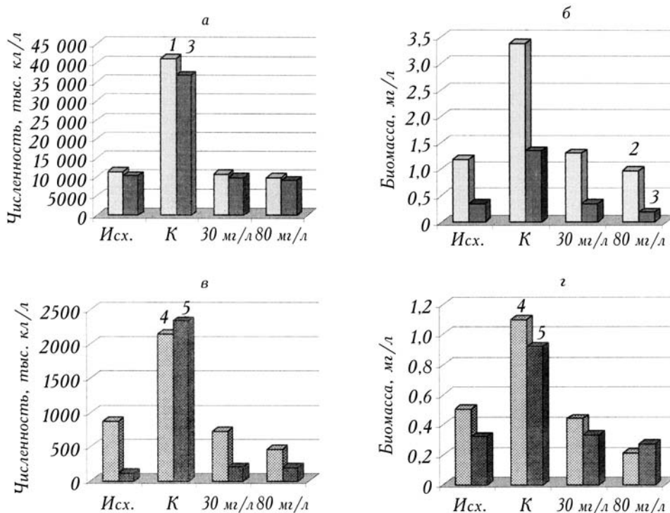
1. Изменение численности (а, в) и биомассы (б, г) планктонных водорослей зал. Оболонь под влиянием фульвокислот на на 5-е сутки опыта: 1 — общая численность; 2 — общая биомасса; 3 — Суанорфита; 4 — Chlorophyta; 5 — Bacillariophyta. Здесь и на рис. 2—5: исх. — исходная, к — контроль.
