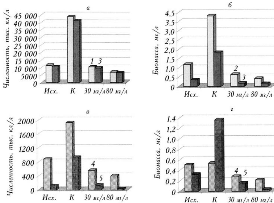
2. Изменение численности (а, в) и биомассы (б, г) планктонных водорослей залива Оболонь под влиянием фульвокислот на 8-е сутки опыта: 1 — общая численность; 2 — общая биомасса; 3 — Суанорхита; 4 — Chlorophyta; 5 — Bacillariophyta.
