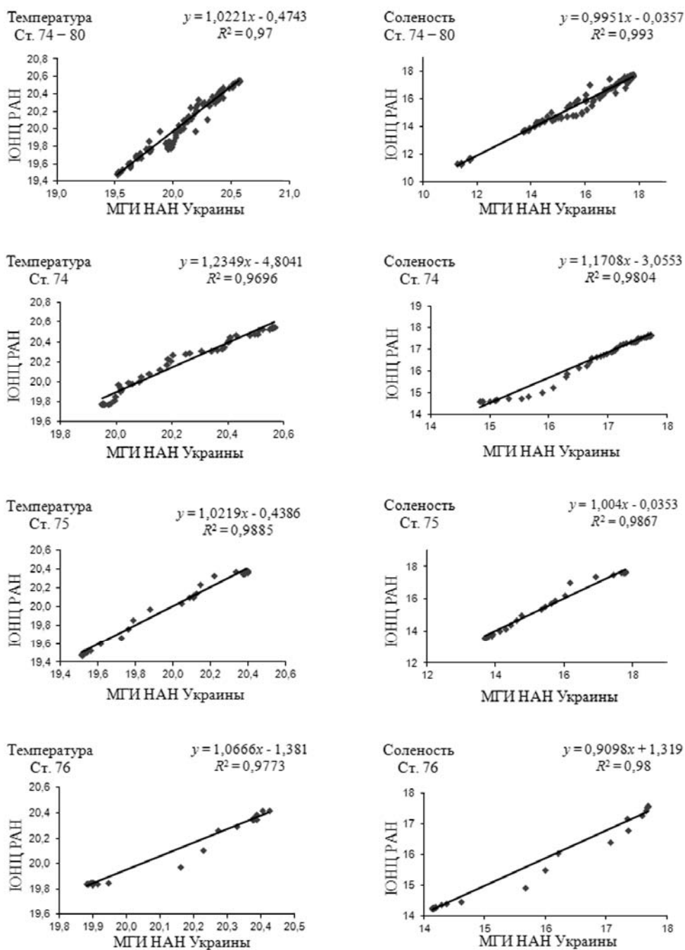
Р и с. 2. Корреляционные зависимости температуры и солености по данным STD-зондов МГИ НАН Украины и ЮНЦ РАН на интеркалибрационных станциях
