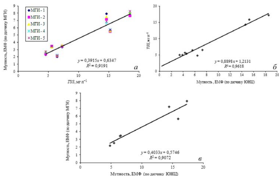
Р и с. 3. Корреляционные зависимости по данным измерения мутности различными средствами
