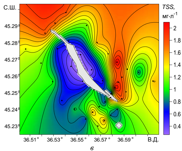
Р и с. 5. Пространственное распределение температуры – a , солености – б и мутности – в в приповерхностном слое (0 ... 1 м) vicinity о. Коса Тузла ISSN 0233-7584. Мор. гидрофиз. журн., 2014, № 1
