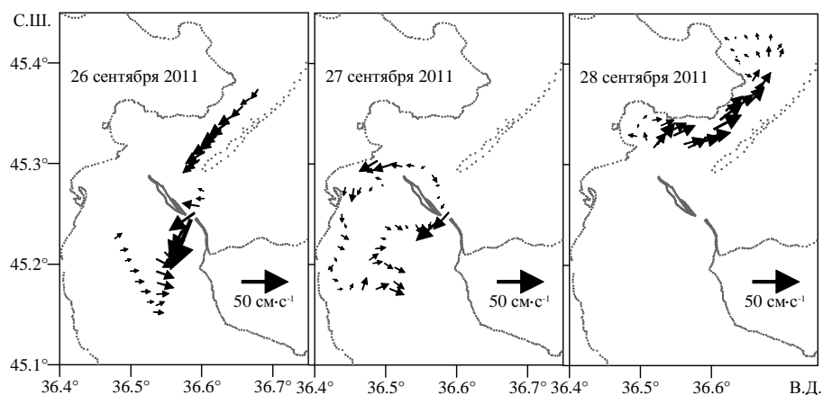
Р и с. 6. Распределение средней по глубине скорости течений
