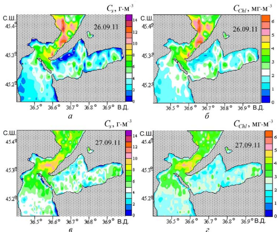
Р и с. 8. Пространственное распределение концентрации взвеси (а, в) и хлорофилла a (б, г) в сентябре 2011 г.
