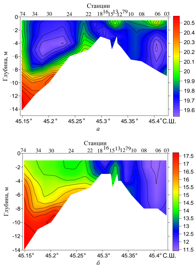
Р и с. 4. Вертикальный разрез по температуре (а) и солёности (б) вдоль Керченского пролива
