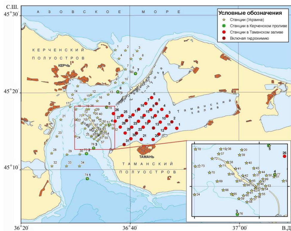
Р и с. 1. Расположение станций при выполнении совместной экспедиции ЮНЦ РАН – МГИ НАН Украины в Керченском проливе
