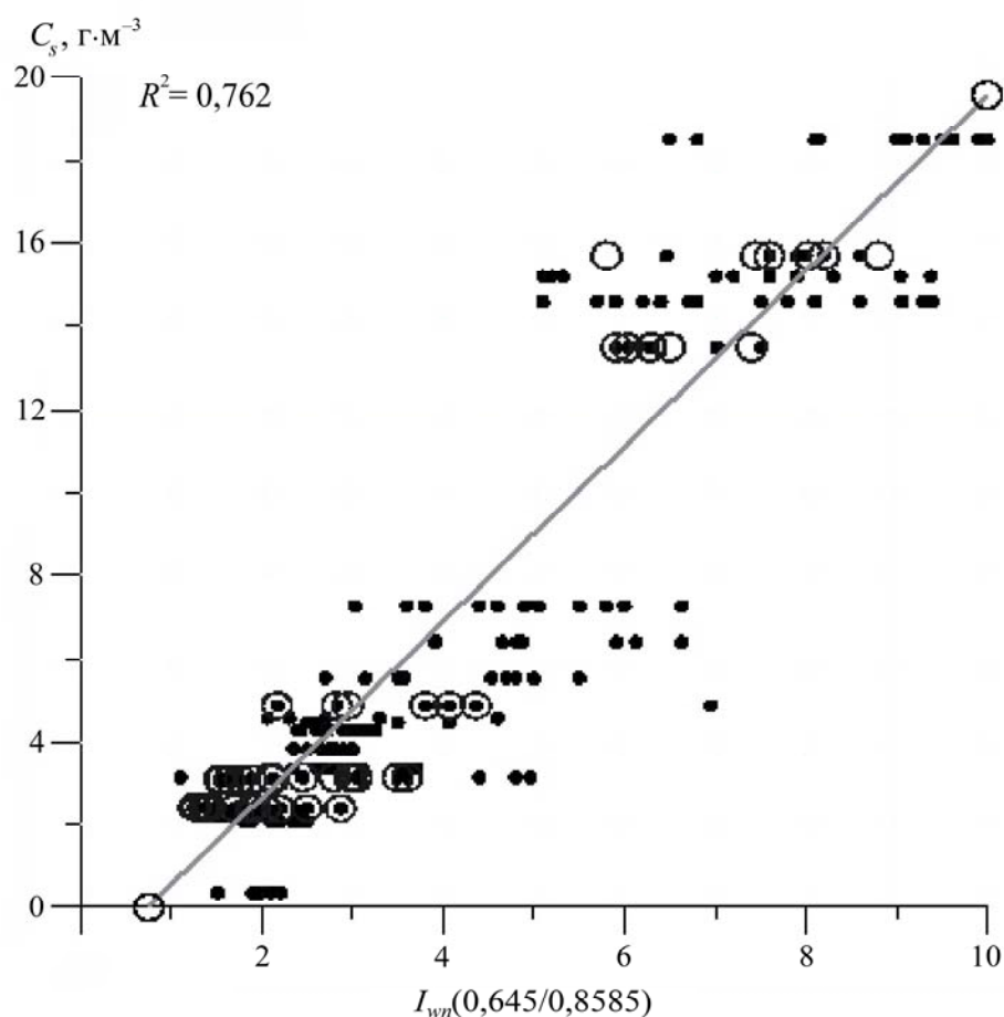
Р и с. 7. Эмпирическая зависимость C_s = f(I_{wm}) по данным совместной экспедиции 26 – 28 сентября 2011 г. (точки) и данным, полученным в 2008 – 2009 гг. (кружки); сплошная линия – регрессионная зависимость
