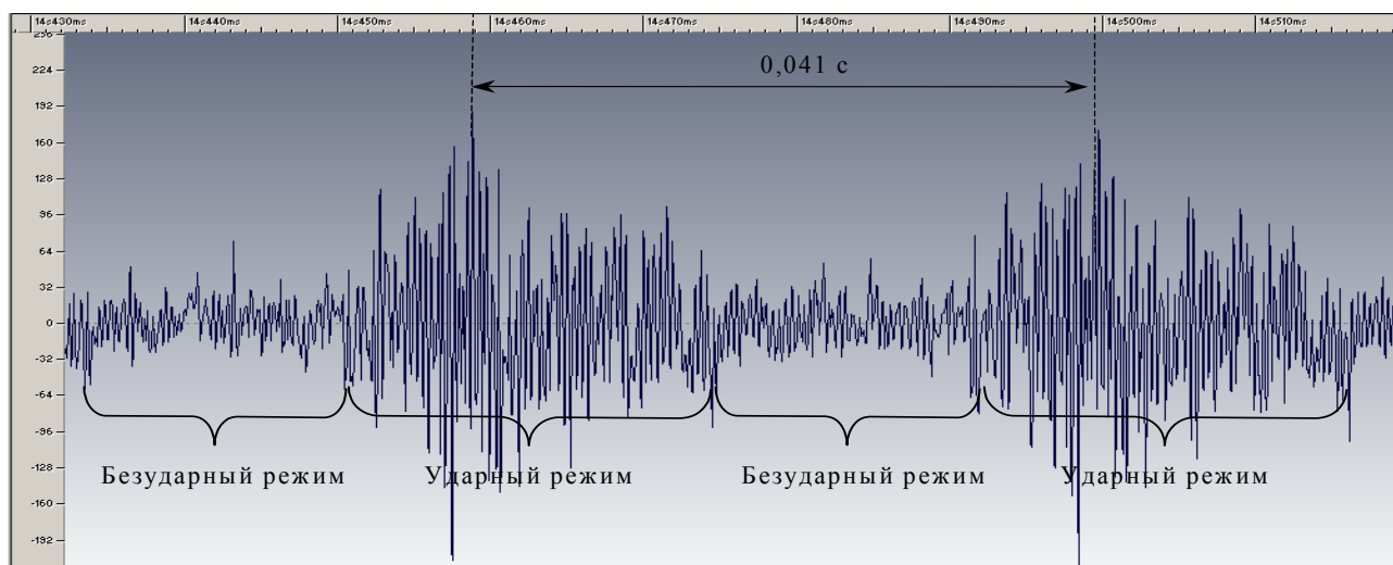
Рисунок 4. Осциллограммы ускорений колебаний ударника грохота
