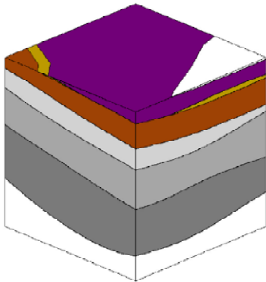
Рис. 11. Аксонометрична проекція (ділянка А)
