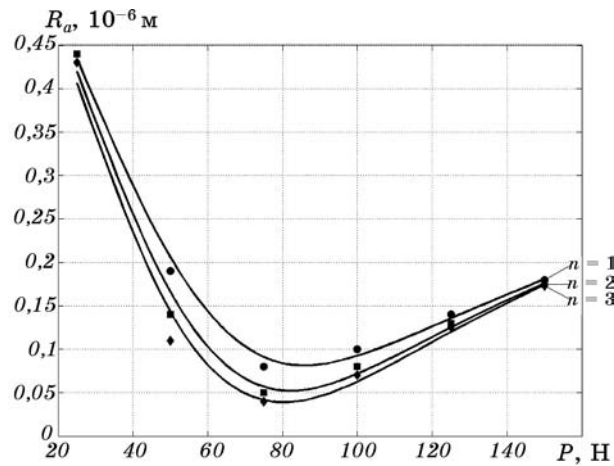
Рис. 5. Зависимость шероховатости поверхности R_a от усилия прижима выглаживателя P при различных количествах проходов для стали 12X18H10T.
