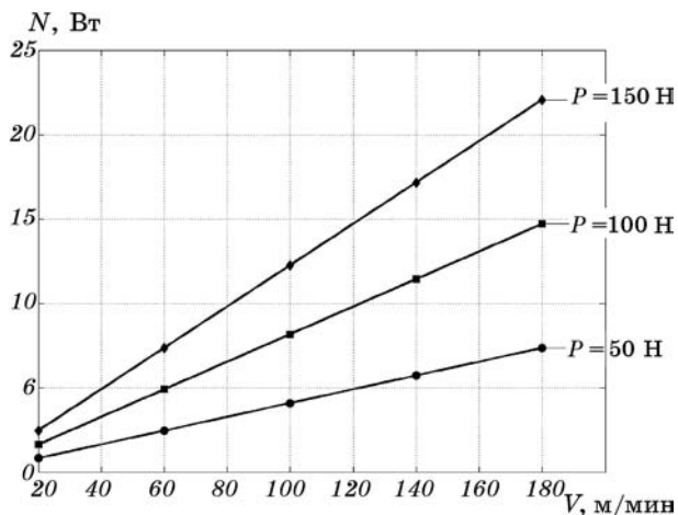
Рис. 10. Зависимость мощности N алмазного выглаживания от скорости выглаживания V для материала 12Х18Н10Т.
