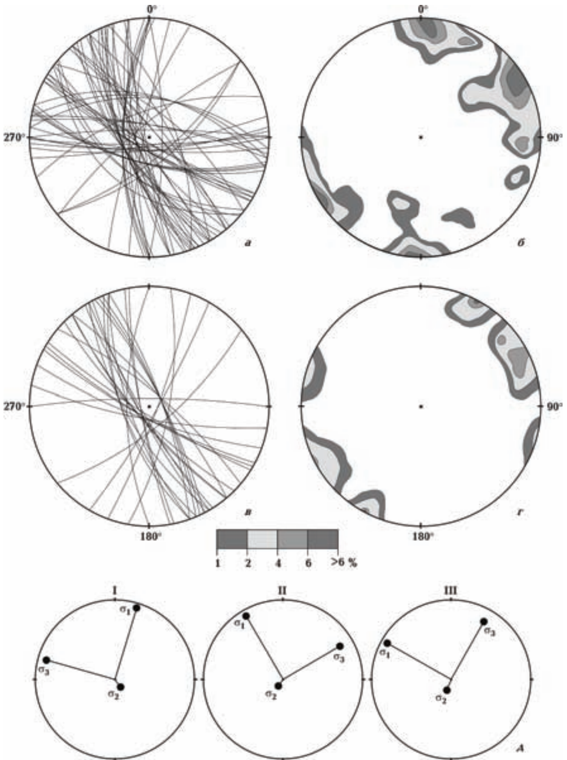
Рис. 3. Структурные S- и \pi S-диаграммы для трещин скалывания (а, б) и отрыва (в, г), а также поля напряжений поздних стадий развития зоны ЗГР (д); \sigma_1 — ось максимального сжатия; \sigma_2 — ось промежуточных напряжений; \sigma_3 — ось максимального растяжения.
