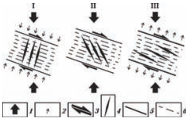
Рис. 4. Реконструкция динамокинематических условий формирования трещин отрыва трех этапов с учетом экспериментальных данных М. В. Гзовского. Схема простого сдвига с дополнительным сжатием (I), без дополнительного сжатия—растяжения (II) и с дополнительным растяжением (III): 1 — направление регионального сжатия; 2 — направление дополнительного сжатия—растяжения; 3 — направления сдвиговых смещений; 4 — структуры растяжения; 5 — границы зоны скалывания; 6 — листоватость зоны скалывания.
