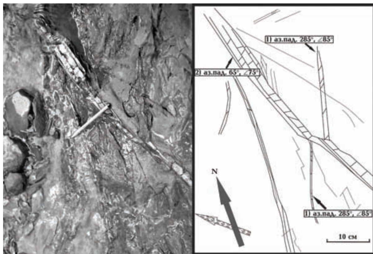
Рис. 2. Фото молодых трещин скалывания и отрыва в пределах обнажения и схематическое изображение взаимоотношений между ними. Стрелками указаны направления на север и разлистования.
