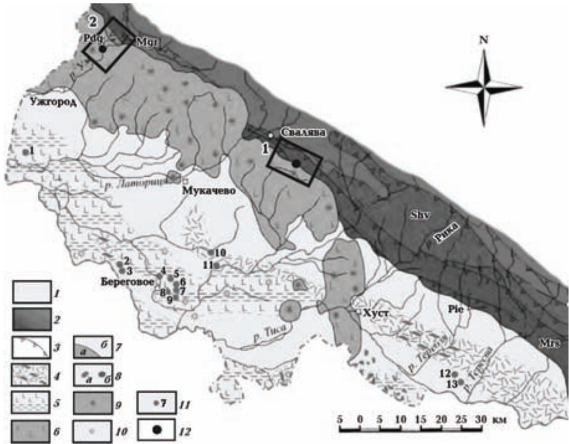
Рис. 1. Расположение кайнозойских магматических пород и вулканических центров в Закарпатском прогибе (Украина) [Павлюк и др., 2013]: 1 — Закарпатский прогиб; 2 — Карпатская скибовая зона; 3 — границы скиб; 4—6 — миоценовые магматические породы (4 — туфы и игнимбриты; 5 — вулканогенно-осадочные породы; 6 — Выгорлат-Гутинский вулканический хребет); 7 — границы разных магматических комплексов (а — на поверхности; б — перекрытые); 8 — интрузии (а — кислого состава; б — основного состава); 9 — магматические центры на поверхности; 10 — перекрытые магматические центры; 11 — расположение скважин; 12 — участки исследований и пункты наблюдений.
