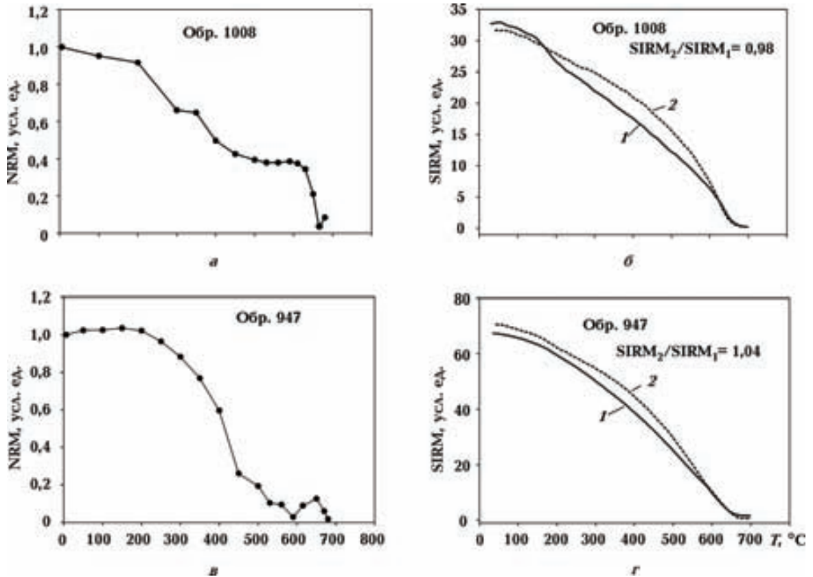
Рис. 6. Примеры температурного размагничивания образцов красноцветов: нормированной NRM в процессе ступенчатого размагничивания (а, в); остаточной намагниченности насыщения (SIRM) в процессе непрерывного нагрева (1 — первый нагрев, 2 — второй нагрев) (б, г).
