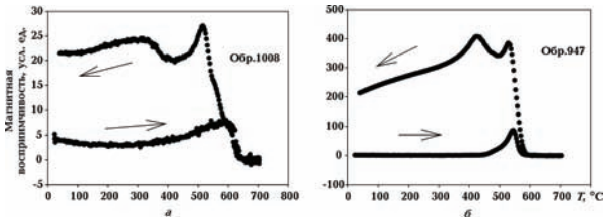
Рис. 7. Изменение магнитной восприимчивости образцов красноцветов в процессе непрерывного нагрева и охлаждения.
