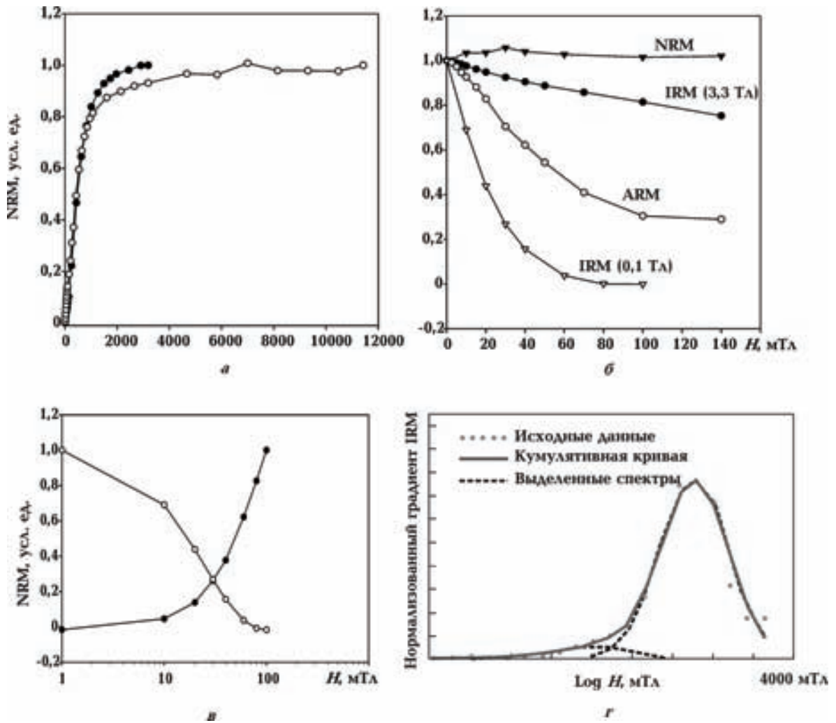
Рис. 8. Кривые насыщения IRM ( а ); кривые размагничивания переменным магнитным полем ( б ): NRM (черные треугольники), IRM наведенной в поле 3,3 Тл (черные круги), ARM (белые круги), IRM наведенной в поле 0,1 Тл (белые треугольники); в — пример сравнения нормализованной кривой IRM и кривой размагничивания IRM, точка пересечения ниже 0,5; г — пример анализа производной кривой IRM по методике [Kruiver et al., 2001].
