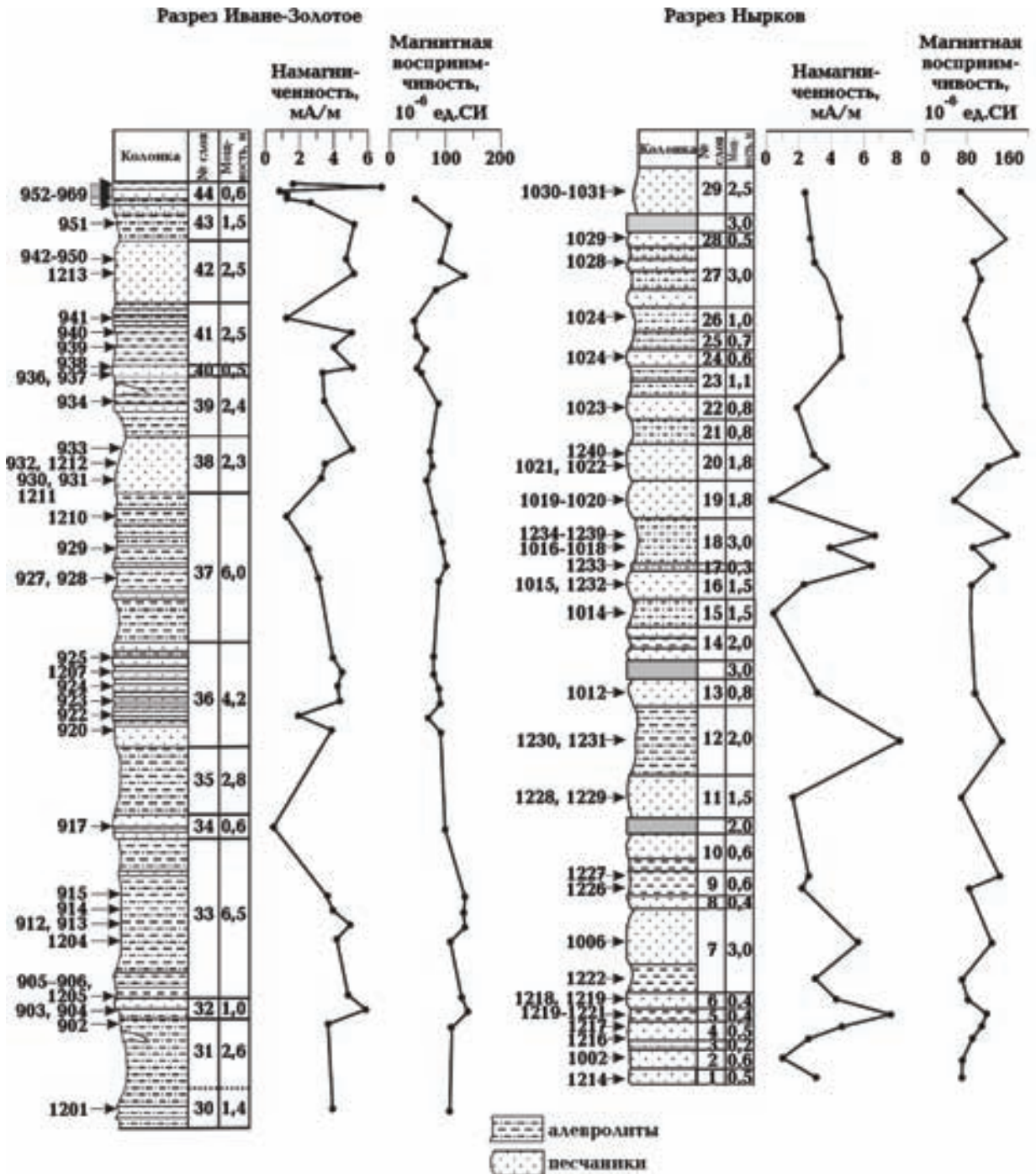
Рис. 2. Палеомагнитные характеристики исследованных разрезов нижнего девона Подолии. Цифры со стрелками — номера и позиции в геологическом разрезе отобранных образцов; номер слоя в соответствии с [Никифорова, Предтеченский, 1968].
