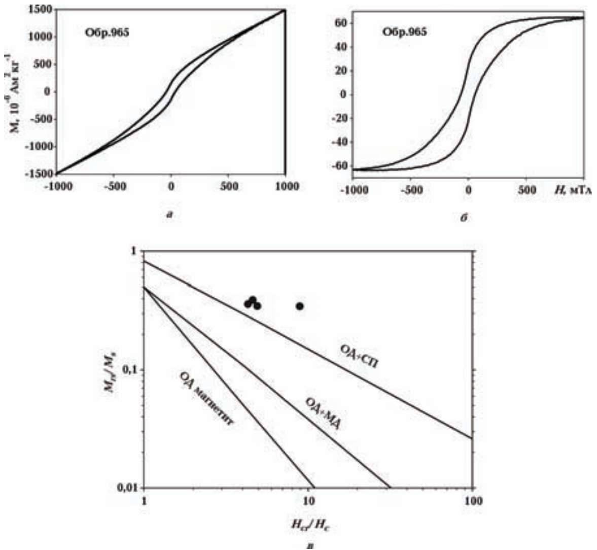
Рис. 9. Примеры петли гистерезиса формы "осиной талии" (а); она же после удаления парамагнитного эффекта (б); соотношение параметров M_{rs} / M_s и H_{cr} / H_c (диаграмма Дзя—Данлопа) (в). Зерна: ОД — однодоменные, МД — многодоменные, СП — суперпарамагнитные.
