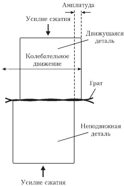
Рис. 1. Схема процесса ЛСТ
