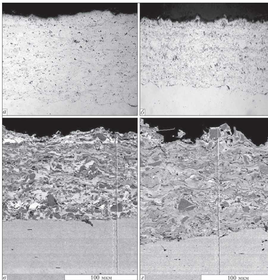
Рис. 3. Микроструктура покрытий из порошков PP-53 (а, в) и PP-53В (б, г) (а, б — микроскоп Неофот, ×400; в, г — электронно-зондовый анализ CamScan)
