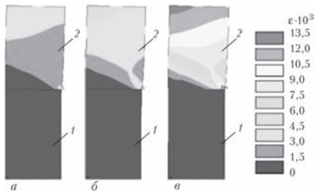
Рис. 2. Изменение эквивалентных пластических деформаций в сечении осесимметричной половины образца при ДС сталей 12Х18Н10Т (1) и 10864 (2) по классической схеме при времени сварки 90 (а), 120 (б), 300 с (в)
