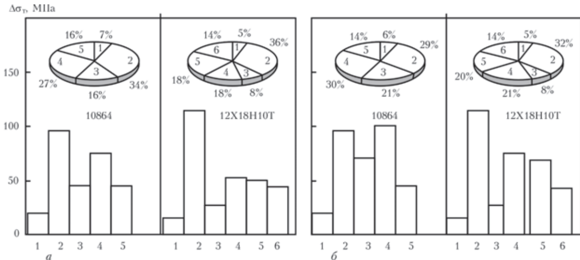
Рис. 6. Влияние структурных факторов на предел текучести металла и долю составляющих в пределе текучести в стыке при ДС по традиционной схеме при постоянной температуре (а) и ДС с термоциклированием (б) в зоне 0: 1 — \Delta\sigma_0 ; 2 — \Delta\sigma_{т.р} ; 3 — \Delta\sigma_3 ; 4 — \Delta\sigma_c ; 5 — \Delta\sigma_d ; 6 — \Delta\sigma_{д.у}
