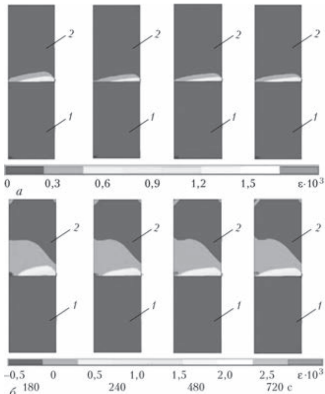
Рис. 3. Изменение полей эквивалентных (а) и сдвиговых (б) пластических деформаций в сечении осесимметричной половины образца при ДС с термоциклированием сталей 12Х18Н10Т (1) и 10864 (2) в течение первого цикла (180, 240 с), после второго (480 с) и после третьего (720 с)
