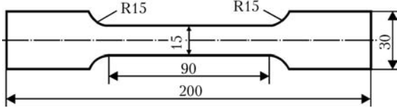
Рис. 2. Схематическое изображение образца для статических испытаний
