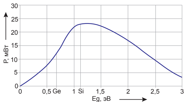
Рис. 1. Зависимость выходной мощности P с 1 \text{ см}^2 от ширины запрещенной зоны
