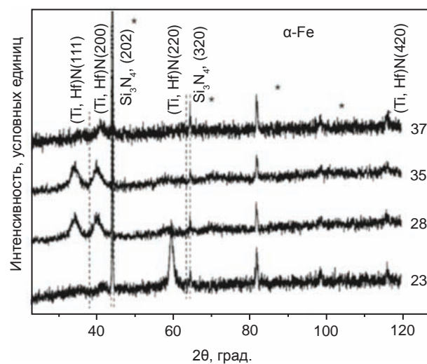
Рис. 6. Дифракционные спектры покрытий, осажденных на стальную подложку при режимах: (23) — -100 В, магнитная сепарация; (28) — -200 В, прямооточный пучок; (35) — -100 В, прямооточный пучок; (37) — -200 В, магнитная сепарация [45]
