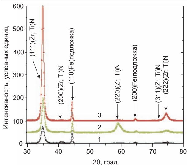
Рис. 1. Участки рентгенограмм покрытий на основе Zr, Ti, Si и N: 1) U_{\text{см}} = -100 В, P = 0,3 Па; 2) U_{\text{см}} = -200 В, P = 0,3 Па, 3) U_{\text{см}} = -200 В, P = 0,7 Па [18]
