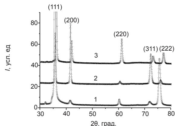
Рис. 1. Участки дифракционных спектров покрытий состава 50 мол. % TiC — 50 мол. % WC, полученных при: 1 — 570 К, 2 — 770 К, 3 — 970 К
