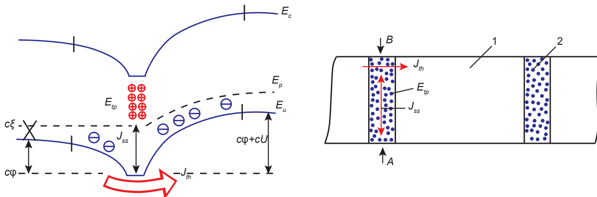
Рис. 2. Зоная диаграмма — а и схема области МЗГ — б; 1 — зерна ПК, 2 — МЗГ
