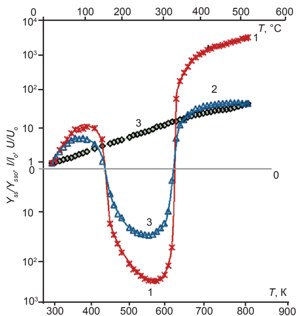
Рис. 1. Относительные изменения темнового тока (1) и напряжения (2), а также проводимости ловушек (3) от температуры на образцах с присутствием щелочных металлов. I_{кзо} , U_{xxo} , Y_{sso} измерены при 300 К
