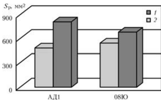
Рис. 2. Площадь растекания S_p припоя системы Al-12Si при флюсовой дуговой (1) и печной (2) пайке
