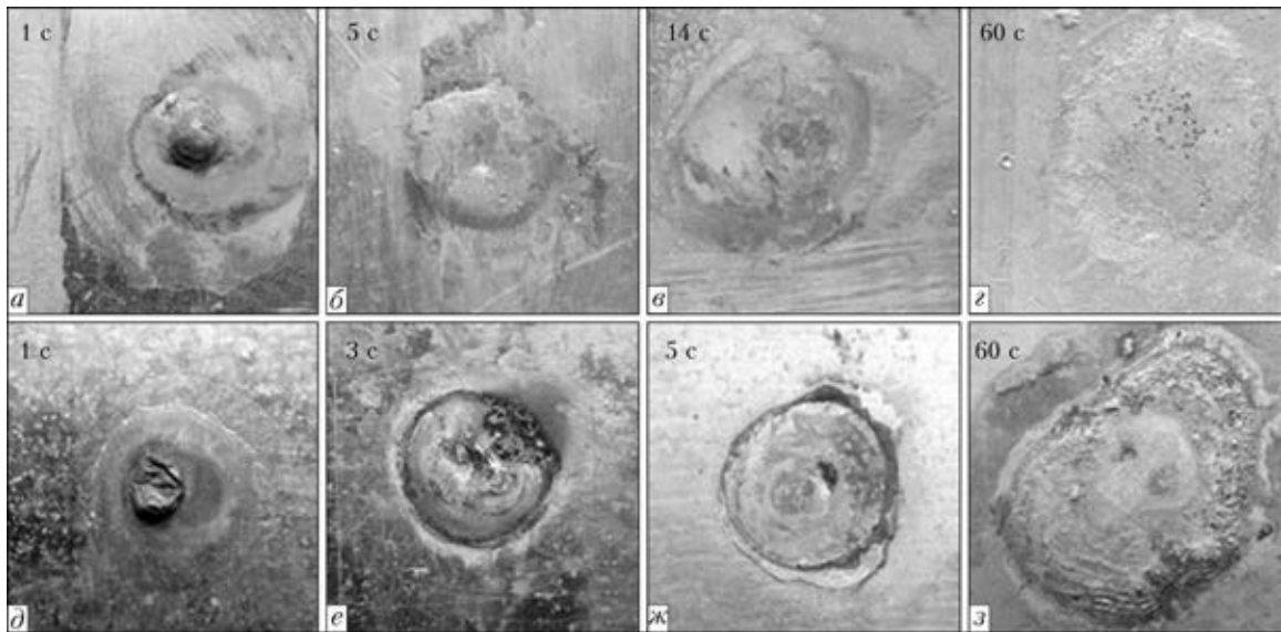
Рис. 1. Капли застывшего припоя системы Al–12Si на алюминии АД1 (а–д) и оцинкованной стали 08Ю (е–з): а–д — АД1; е–ж — сталь 08Ю (дуговая пайка в аргоне, I_{п} = 25 А, T_{п} = 600...615 °С, аппарат MASTERTIG MSL™ 2300 ACDC фирмы «Kemppi», Финляндия); з — сталь (печная пайка в азоте, T_{п} = 600 \pm 3 °С)
