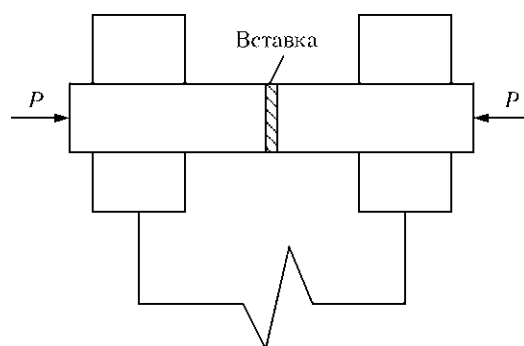
Рис. 1. Схема сварки сопротивлением с использованием композитной вставки
