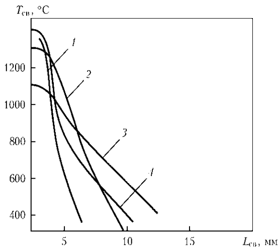
Рис. 2. Распределение температуры сварки T_{св} перед осадкой при контактной сварке арматуры диаметром 32 мм непрерывным оплавлением (1), с композитной вставкой (2), сопротивлением (3), оплавлением с подогревом (4) ( L_{св} — расстояние от зоны сварки)
