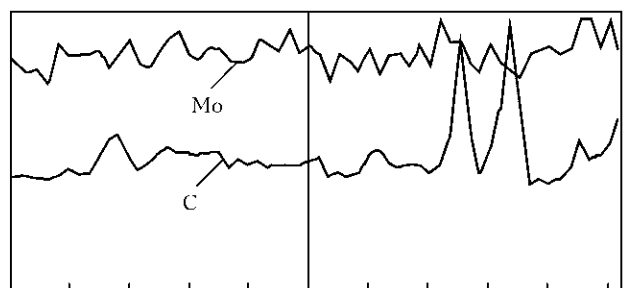
Рис. 5. Распределение углерода и молибдена поперек сварного шва, выполненного на стали 25Г2С (база измерения 120 мкм с шагом 2 мкм)
