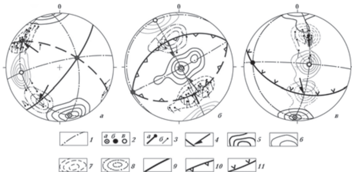
Рис. 3. Стереографическое отображение СКП тектонических разрывов и смещений, сформированных в условиях различных деформационных режимов — сдвигового (а), сбросового (б) и взбросового (в); пункты наблюдений и номера парагенезисов (указаны в скобках) соответственно Kastel (1), Iograf (1) и Balakl_1(1): 1, 2 — проекции плоскостей (1) и главных осей (2) нормальных напряжений (а — \sigma_1 , б — \sigma_2 , в — \sigma_3 ); 3 — полюсы разрывов и направления подвижек (а — по парагенезису в целом, усредненные значения, б — по отдельным зеркалам скольжения); 4 — проекция усредненно-го вектора смещения по парагенезису (определена по максимуму плотностей проекций единичных векторов каждой системы); 5—8 — изолинии плотностей по совокупности замеров «квазиглавных» осей нормальных напряжений \sigma_1 (5), \sigma_3 (6), полюсов (7) и проекций векторов смещений (8); 9—11 — проекции плоскостей и характеристика структурно-кинематических типов разрывов (9 — сдвиг, 10 — сбросов, 11 — взбросов, сплошные — основные, пунктирные — слабовыраженные).
