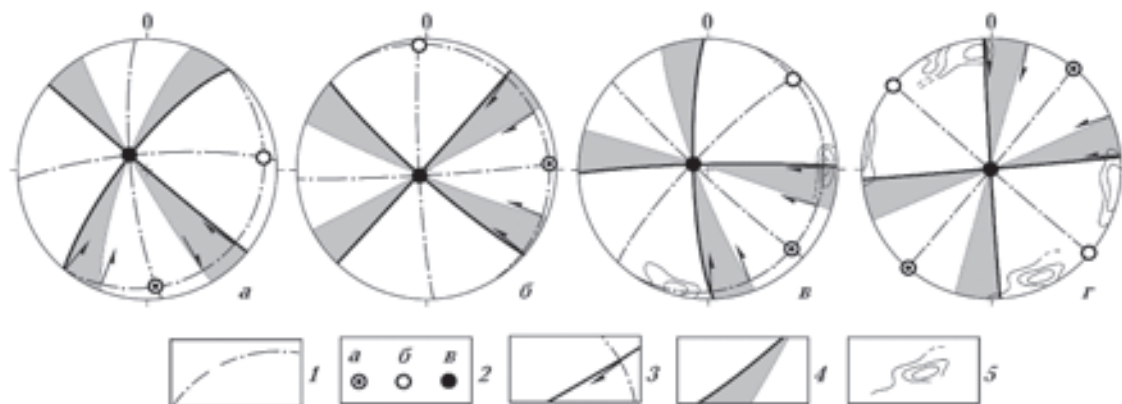
Рис. 9. Стереографические модели сдвиговых деформационных режимов, обусловивших процессы новейшего тектонического разрывообразования в пределах Горного Крыма: а — субмеридионального сжатия—субширотного растяжения; б — субмеридионального растяжения—субширотного сжатия; в — юго-восточного сжатия—северо-восточного растяжения; г — юго-западного сжатия—юго-восточного растяжения: 1—2 — проекции плоскостей (1) и главных осей (2) нормальных напряжений (а — \sigma_1 , б — \sigma_2 , в — \sigma_3 ); 3 — проекции векторов смещений; 4 — секторы наиболее вероятного разрывообразования; 5 — некоторые соответствующие им максимумы в изолиниях плотностей полюсов разрывов (остальные пояснения см. в тексте).
