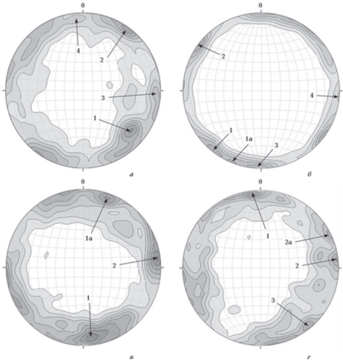
Рис. 8. Сводные стереограммы полюсов разрывов (а), проекций векторов смещений (б) и главных осей напряжений \sigma_1 (в) и \sigma_3 (г) для зеркал скольжения СКП, сформированных в условиях сдвиговых деформационных режимов.
