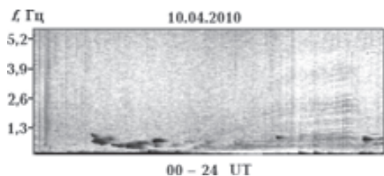
Рис. 5. Периодическая полосовая структура электромагнитного шумового излучения как проявление одновременно ионосферного (широкие полосы) и надionoсферного (узкие полосы) резонаторов. Обсерватория Монды.
