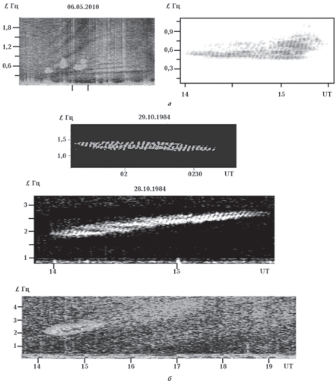
Рис. 4. Пример серий жемчужин: а — обсерватория Монды; б — обсерватория Борок: верхняя панель — геомагнитные пульсации типа Pc1 (жемчужины), наблюдавшиеся в утренние часы местного времени (LT=UT+3); средняя и нижняя панели — пульсации, наблюдавшиеся в вечернее время; заметна дискретизация по частоте, на нижней панели видны наклонные полосы, характерные для ионосферных альвеновских резонансов.
