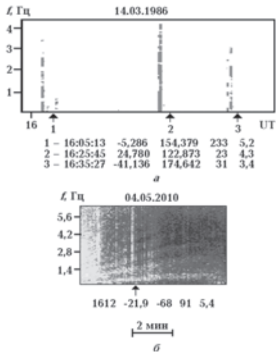
Рис. 7. Импульсы, связанные с подготовкой землетрясений: а — обсерватория Борок; б — обсерватория Монды. Цифры под рисунками означают следующее: время сейсмического толчка (UT), координаты эпицентра (географические широта и долгота), глубина очага, магнитуда.
