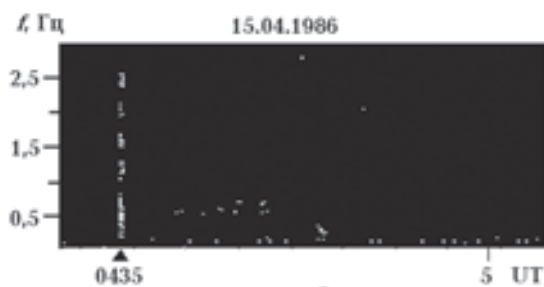
Рис. 5. Периодическая полосовая структура электромагнитного шумового излучения как проявление одновременно ионосферного (широкие полосы) и надionoсферного (узкие полосы) резонаторов. Обсерватория Монды.
