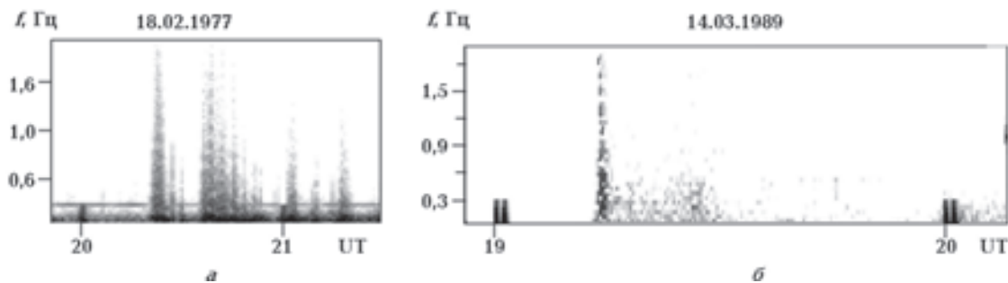
Рис. 1. Пример появления дискретной структуры в спектре широкополосного всплеска иррегулярных колебаний Pi1B. Обсерватория Борок.
