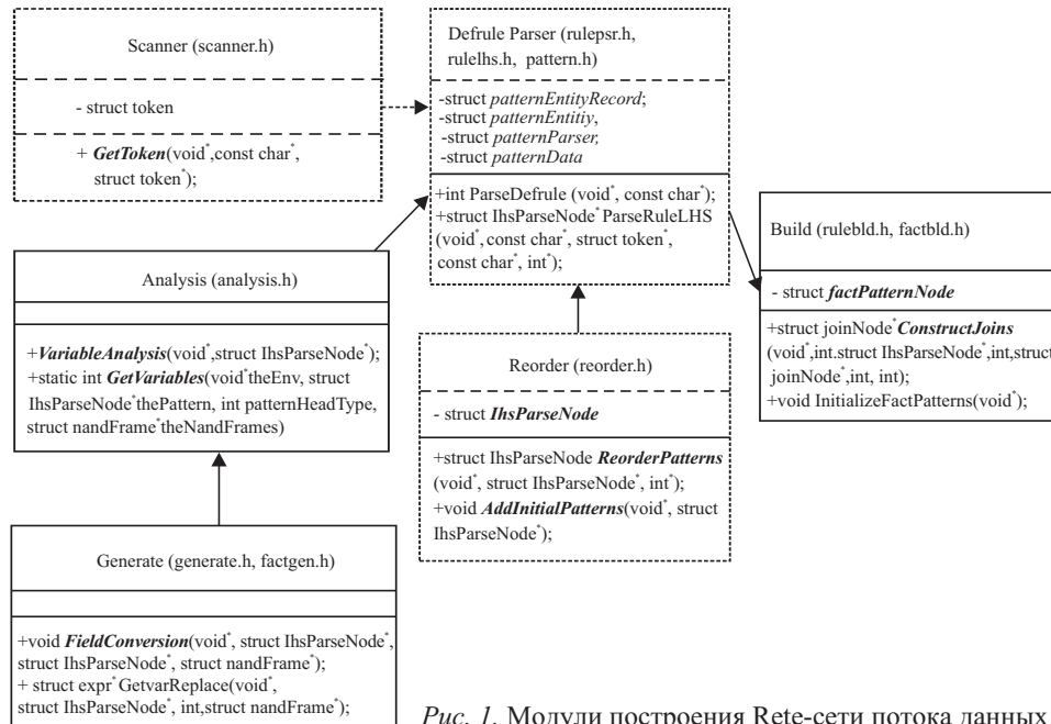
Рис. 1. Модули построения Rete-сети потока данных
