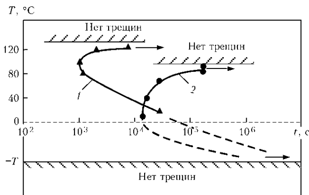
Рис. 7. Обобщенные термокинетические кривые замедленного разрушения сварных соединений мартенситной 10X9MFB (1) и бейнитной 10ГН2МФА (2) сталей при \sigma = 320 МПа
