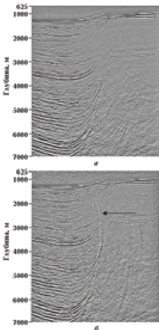
Рис. 8. Изображения соляного штока в Мексиканском заливе, полученные с помощью преломляющей миграции Кирхгофа без учета (а) и с учетом (б) рефракционированных волн. Стрелка указывает на улучшенное изображение стенки штока после учета рефракции.
