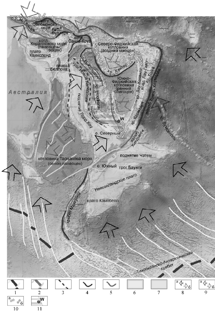
Фрагмент крупного офиолитового покрова: 1 – современные оси спрединга и трансформные разломы; 2 – древние (неактивные) оси спрединга и трансформные разломы; 3 – рифтовые трого; 4 – глубоководные желоба; 5 – зоны обдукции и коллизийные сuture; 6 – области с континентальной земной корой; 7 – океаническая кора окраинных морей; 8 – современные (а) и древние (б) направления транзитных движений плит; 9 – направления субдукционных (а) и обдукционных (б) движений; 10 – вулканы современные (а) и неогеновые (б); 11 – вольфрамовое проявление Мотукоако и возможные контуры вольфрамоносных провинций региона. Геоморфологическая основа: http://data.gns.cri.nz/geoatlas/text.jsp?Page=2
