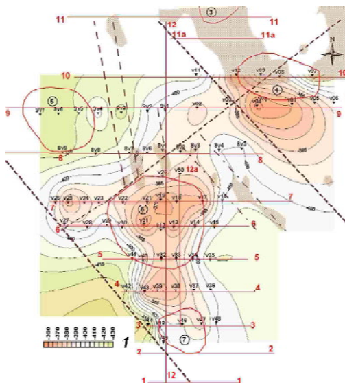
Рис. 3. Карта глубин подошвы зоны мерзлоты лицензионного участка: 1 – шкала значений глубины подошвы зоны мерзлоты, м. Остальные условные обозначения см. на рис. 1
