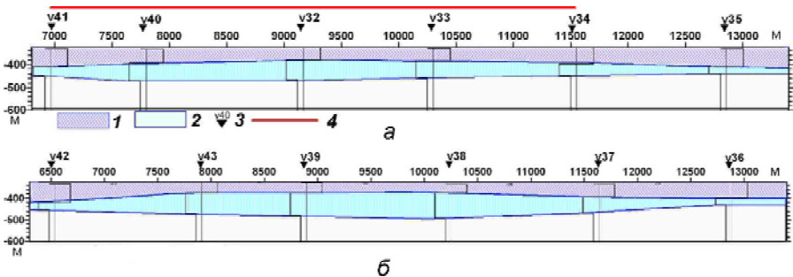
Рис. 5. Характер изменения мощностей многолетнемерзлых пород и талых вод вдоль профилей зондирования ВЭРЗ № 5 (а) и № 4 (б): 1 – слой многолетнемерзлых пород; 2 – толщина талых вод; 3 – пункт ВЭРЗ; 4 – положение выделенных по сейсмическим данным структурных поднятий на профилях зондирования
