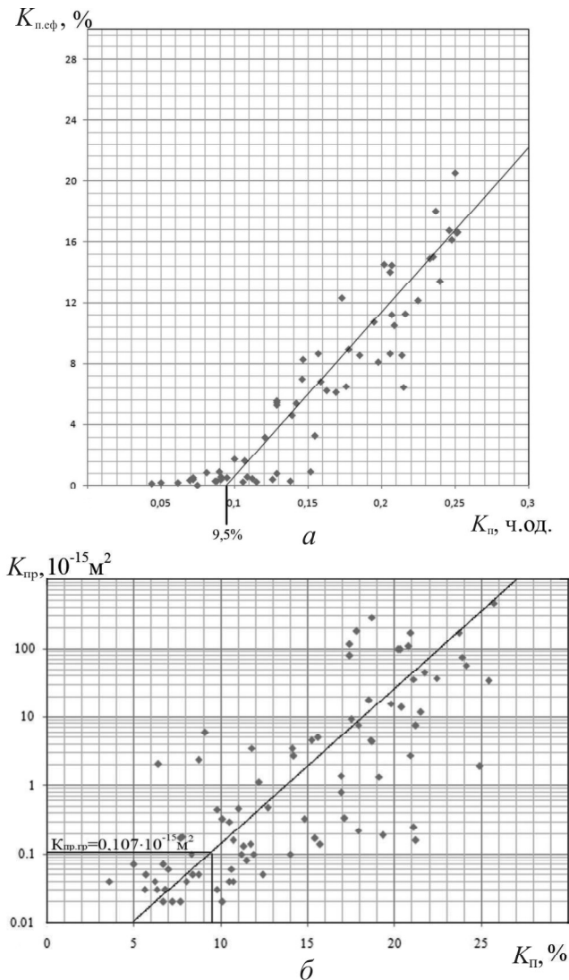
Рис. 4. Зіставлення коефіцієнта пористості з K_{п.эф} (а) і K_{п} (б)
