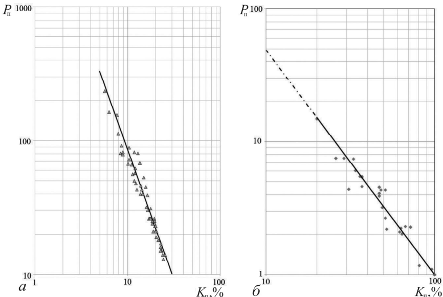
Рис. 1. Залежності P_{\Pi} = f(K_{\Pi}) (а) і P_{\Pi} = f(K_{\text{в}}) (б)
