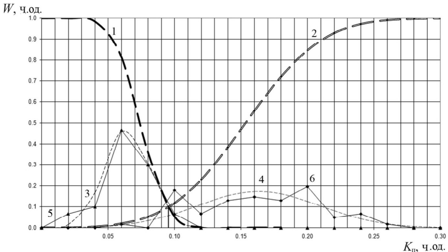
Рис. 3. Визначення граничного значення відкритої пористості, криві розподілу: 1 – неколектор, кумулянта; 2 – колектор, кумулянта; 3 – неколектор, теоретична; 4 – колектор, теоретична; 5 – неколектор, фактична; 6 – колектор, фактична.
