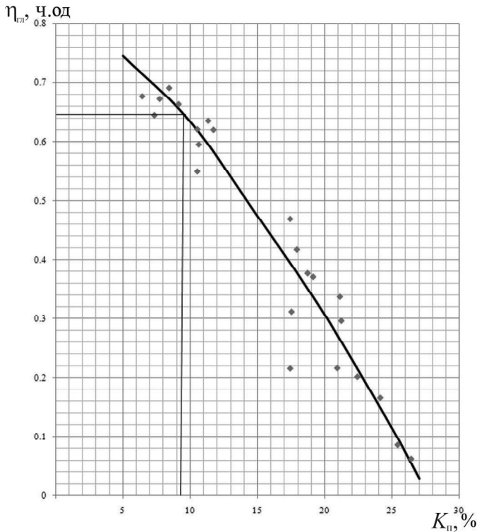
Рис. 7. Зіставлення параметрів K_{п} та \eta_{гл}
