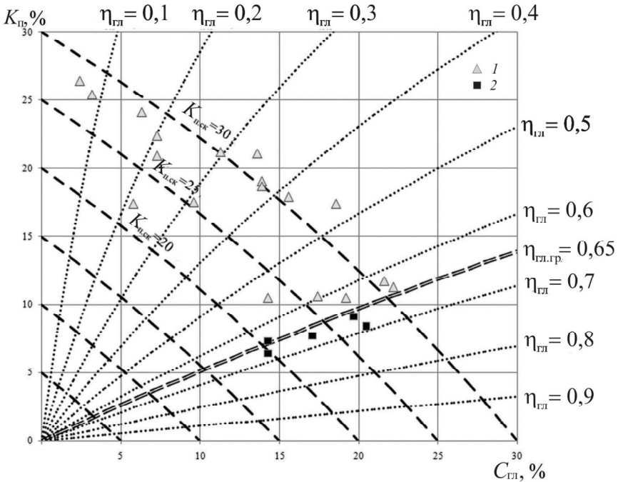
Рис. 6. Зіставлення параметрів K_{п} та C_{гл} : 1 – колектор; 2 – неколектор
