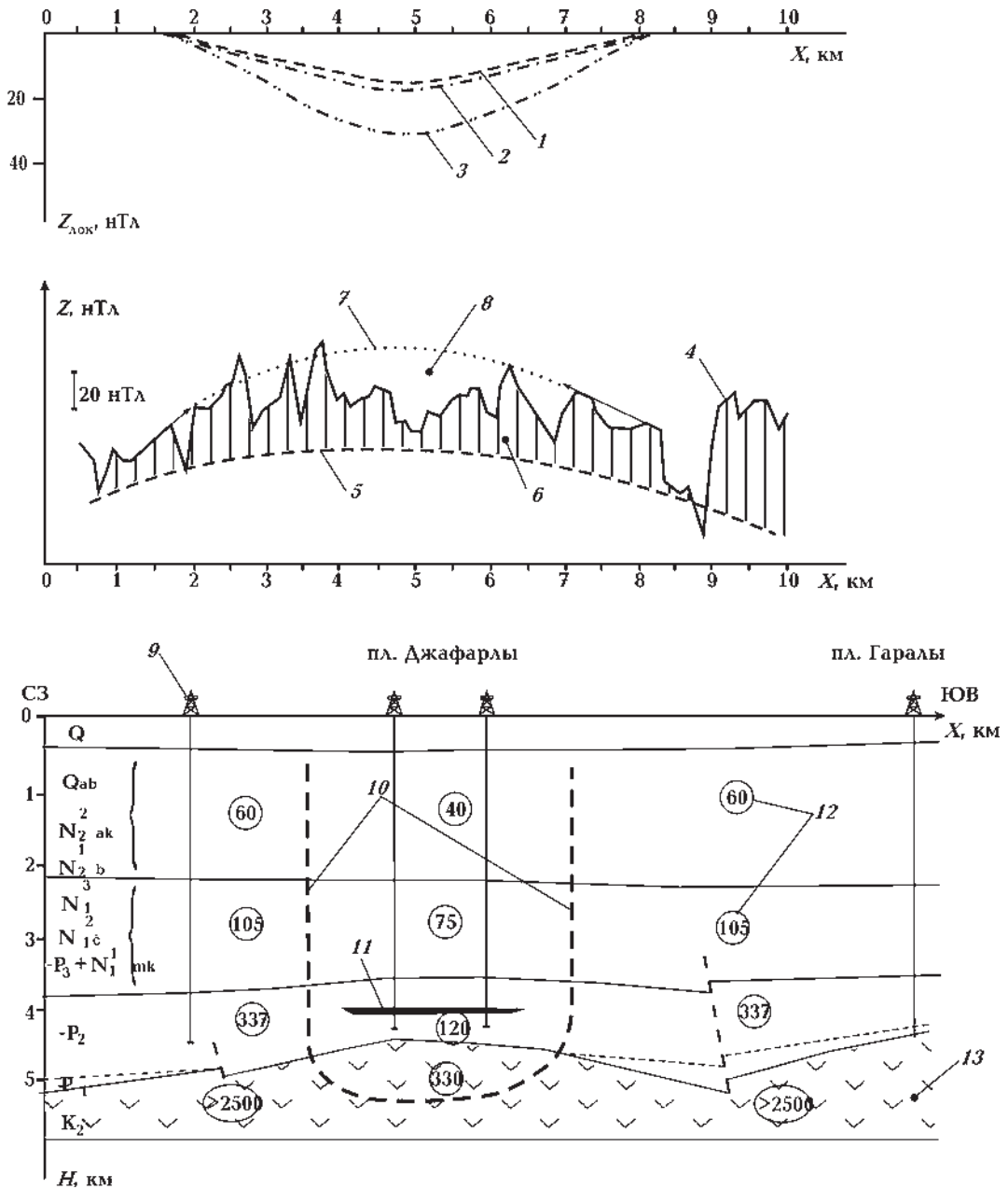
Рис. 2. Геоматнитное моделирование на пл. Джафарлы (юго-восточная часть Среднекуриинской впадины). Условные обозначения см. на рис. 1.
