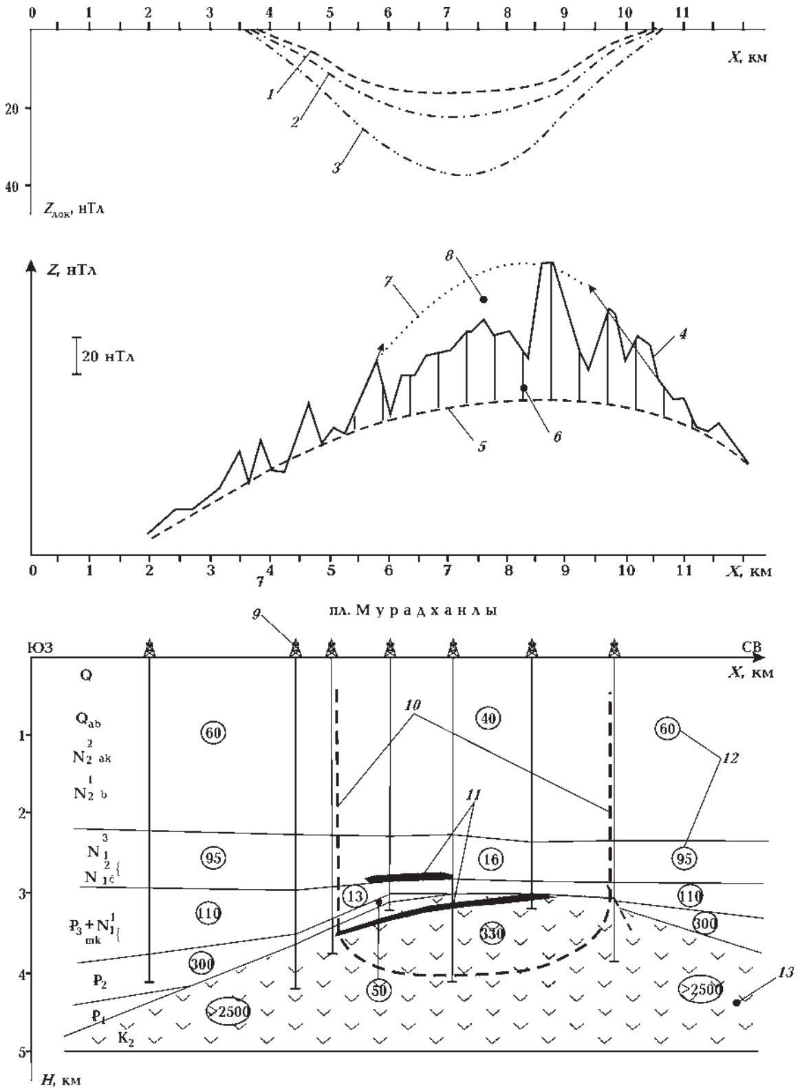
Рис. 1. Геомагнитное моделирование на пл. Мурадханлы (юго-восточная часть Среднекуринской впадины). Вычисленные геомагнитные эффекты субвертикальной зоны: 1 — над залежью; 2 — под залежью; 3 — всей субвертикальной зоны; 4 — наблюдаемая кривая магнитного поля; 5 — региональный фон; 6 — локальный максимум; 7 — восстановленный максимум; 8 — локальный минимум; 9 — глубокие скважины; 10 — границы субвертикальной залежной зоны; 11 — залежь нефти; 12 — осредненные значения магнитной восприимчивости по горизонтам ( 60 \cdot 10^{-6} СГС); 13 — эффузивные образования.
