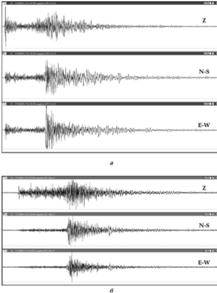
Рис. 1. Примеры цифровых записей землетрясений по составляющим Z, N—S, E—W: а — 5 октября 2007 г., K_{\Pi} = 12,7 ; станция "Симферополь"; б — 17 марта 2011 г., K_{\Pi} = 10,8 , станция "Ялта".
