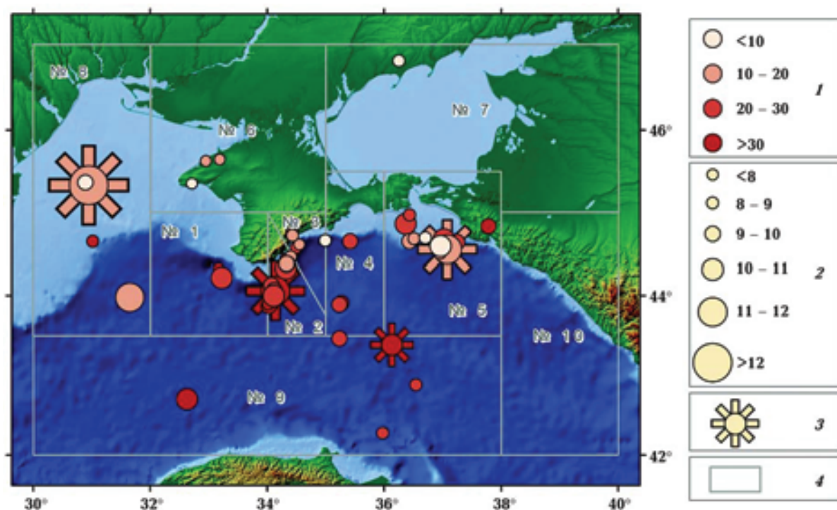
Рис. 2. Карта эпицентров землетрясений Крыма, для которых восстановлены очаговые параметры: 1 — глубина очагов, км, 2 — энергетический класс K_{\Gamma} , 3 — землетрясения с известными механизмами очагов, 4 — границы сейсмоактивных районов с указанием их номеров [Пустовитенко и др., 1989]: № 1 — Севастопольский, № 2 — Ялтинский, № 3 — Алуштинский, № 4 — Судакско-Феодосийский, № 5 — Керченско-Анапский, № 6 — Степной Крым, № 7 — Азово-Кубанский, № 8 — Северо-Западный, № 9 — Черноморская впадина, № 10 — Восточный.
