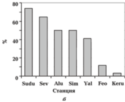
Рис. 3. Распределения количества: a — землетрясений по сейсмическим районам; б — записей сейсмических станций, использованных в оценке очаговых параметров.
