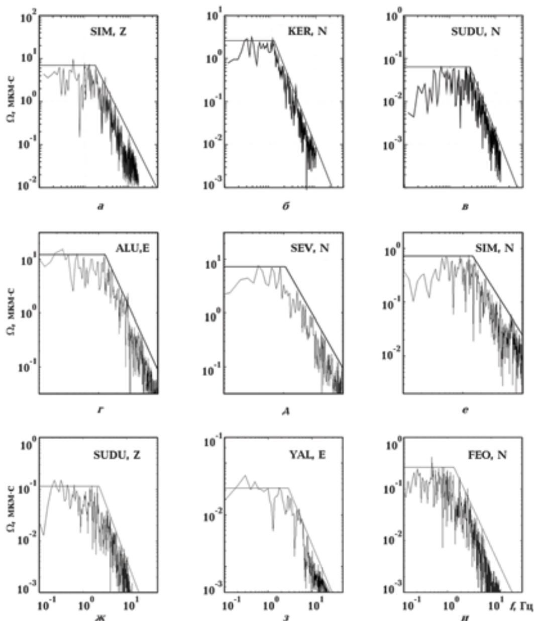
Рис. 4. Примеры амплитудных спектров объемных сейсмических волн землетрясений Крыма: а — № 4, 07.05.2008; б — № 6, 24.07.2008; в — № 8, 22.09.2008; г — № 16, 12.04.2009; д — № 16, 24.04.2010; е — № 19, 18.04.2009; ж — № 30, 24.07.2010; з — № 37, 06.11.2010; и — № 38, 06.11.2010. Номера землетрясений и даты соответствуют таковым в табл. 1.
