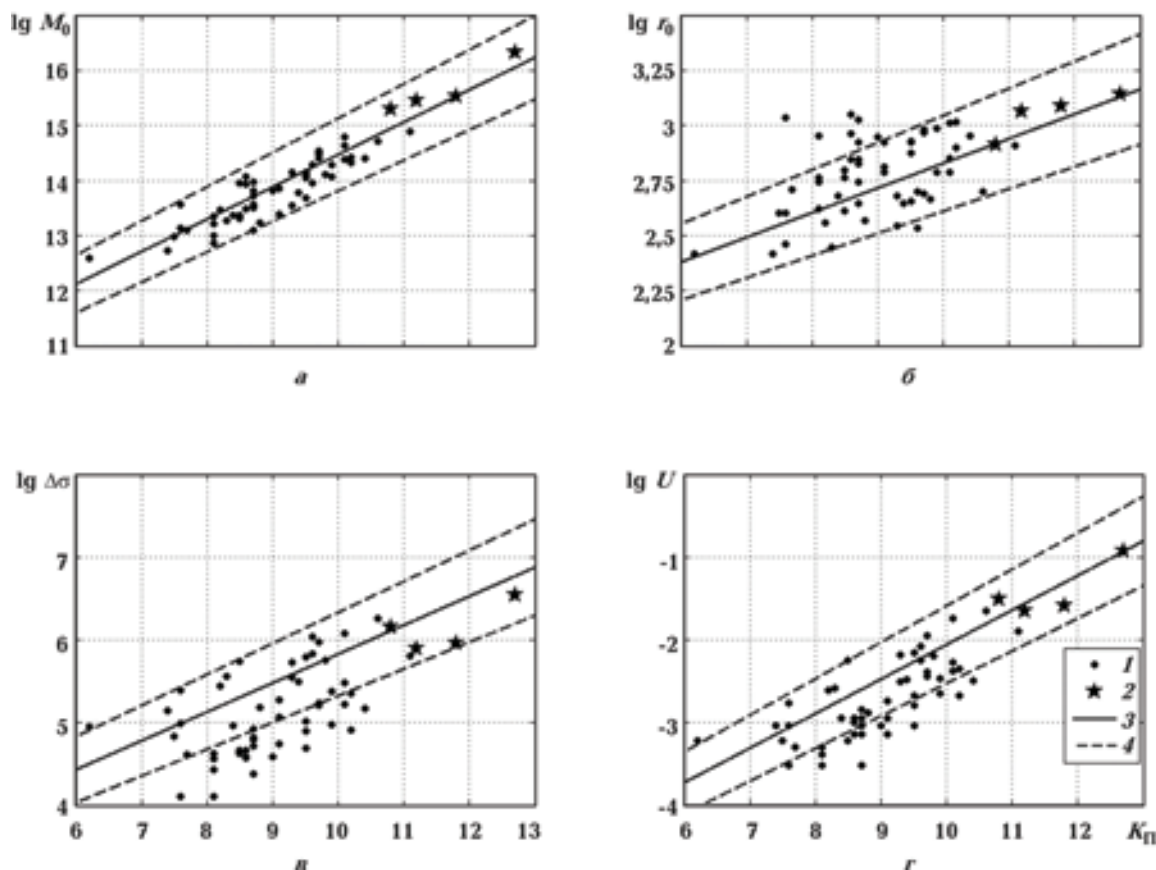
Рис. 5. Зависимости динамических параметров очагов землетрясений Крыма от энергетического класса K_{\Pi} : а — сейсмического момента M_0 ; б — радиуса дислокации r_0 ; в — сброшенного напряжения \Delta\sigma ; г — средней подвижки по разрыву \bar{U} ; 1 — индивидуальные значения параметров по цифровым записям; 2 — значения параметров землетрясений, для которых определен механизм очага; 3 — долговременные зависимости (1)–(4); 4 — доверительный интервал.
