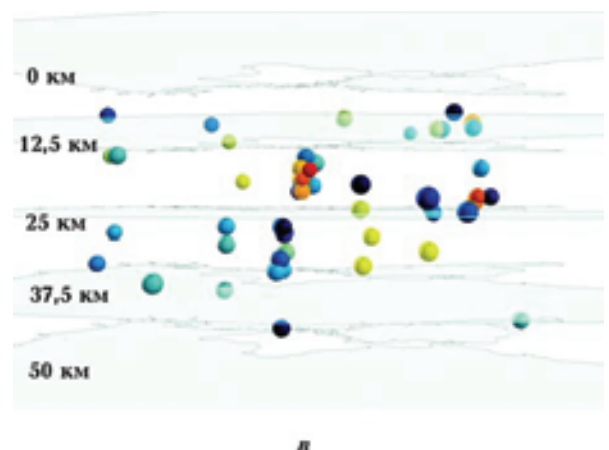
Рис. 6. Пространственное распределение \delta \lg X очаговых параметров: a — средней подвижки по разрыву \bar{U} ; б — сброшенного напряжения \Delta\sigma ; в — распределение \delta \lg \Delta\sigma по глубине.
