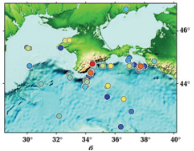
Рис. 3. Распределения количества: a — землетрясений по сейсмическим районам; б — записей сейсмических станций, использованных в оценке очаговых параметров.
