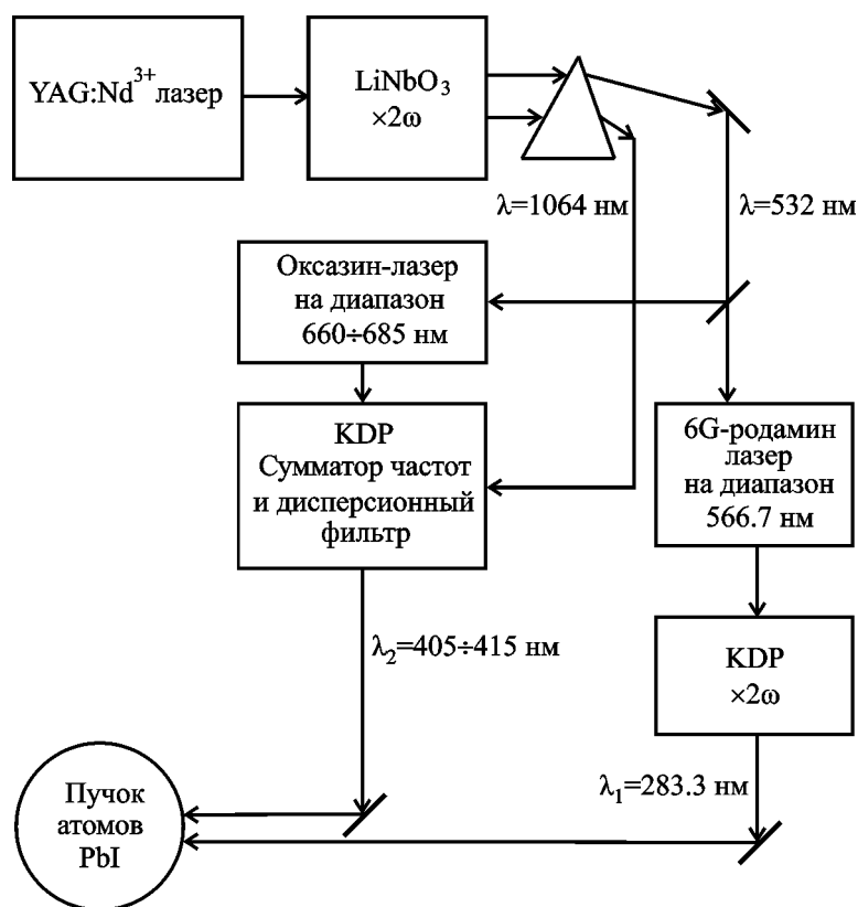
Рис. 2. Схема оптической части спектрометра для исследований nP состояний атомов свинца
