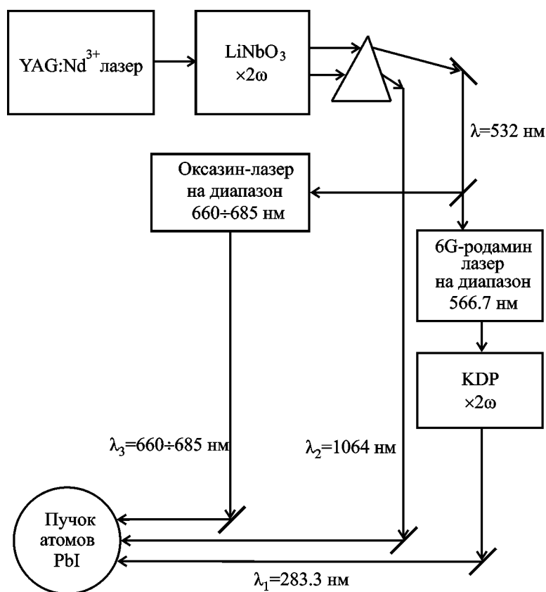
Рис. 4. Схема оптической части спектрометра для исследований nS и nD состояний атомов свинца
