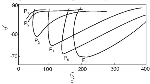
Рис. 1. Зависимость фазы ВЧ тока \vartheta от приложенного к ВЧЕ разряду напряжения U_0 при различных давлениях азота N_2 . Расстояние между электродами l = 54 \text{ мм} ; P_1 = 3 \cdot 10^{-2} \text{ Тор} ; P_2 = 8 \cdot 10^{-2} \text{ Тор} ; P_3 = 2,2 \cdot 10^{-1} \text{ Тор} ; P_4 = 6 \cdot 10^{-1} \text{ Тор} ; P_5 = 1,4 \text{ Тор} ; P_6 = 2 \text{ Тор} .
