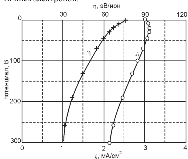
Рис. 18. График зависимости плотности тока ионов j_i и энергетической цены иона \eta от ВЧ потенциала на электроде при постоянном параметрическом давлении pd = 3 \cdot 10^{-3} Торр·см и постоянной суммарной мощности W , нормированной на единицу поверхности ( P/S = 0,25 Вт/см 2 ). Рабочий газ – аргон.
