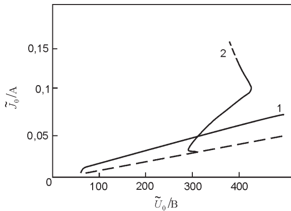
Рис. 2. Статические реактивные ВАХ ВЧЕ разряда в \alpha - и \gamma -режимах. Рабочий газ – N_2 , расстояние между электродами l = 54 мм; Давление газа P_1 = 6 \cdot 10^{-2} Тор; P_2 = 5,5 \cdot 10^{-2} Тор. Пунктирная прямая – величина ВЧ тока конденсатора в отсутствии разряда.
