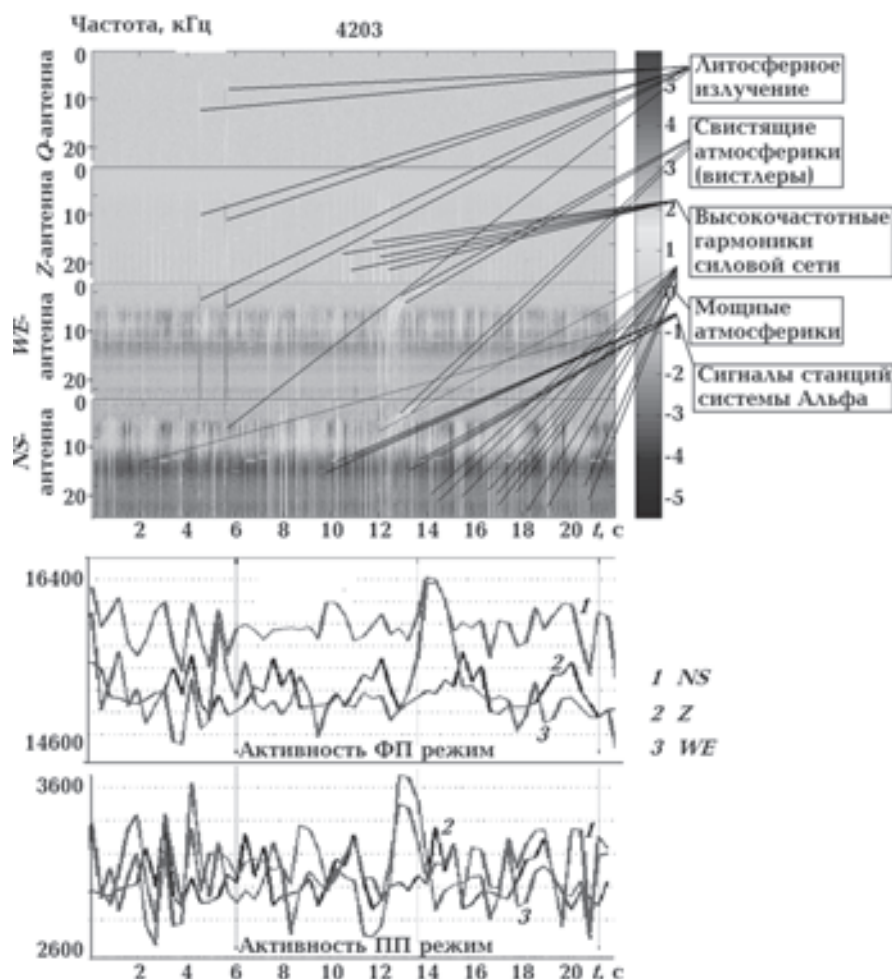
Рис. 6. Четырехканальная спектрохронограмма и сформированная из нее «активность».
