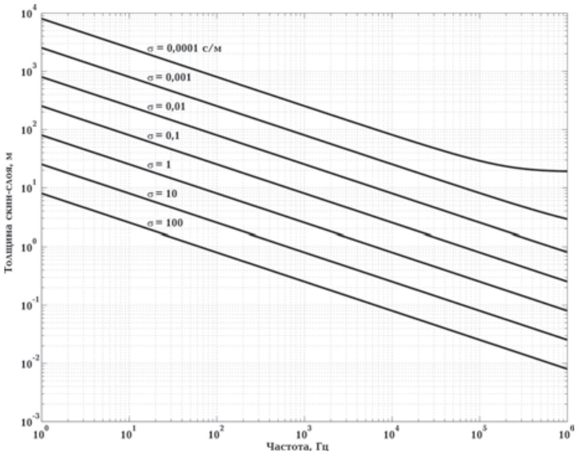
Рис. 2. Зависимость величины скин-слоя от частоты и проводимости среды.
