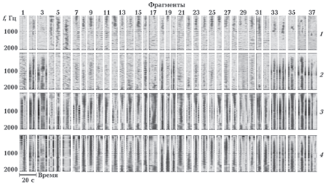
Рис. 7. Коллекция всплесков литосферного происхождения.
