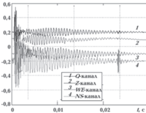
Рис. 5. Волновые формы сигналов литосферного излучения.
