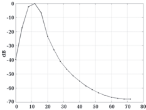
Рис. 4. Зависимость величины сигнала квадрупольной антенны от расстояния до источника.
