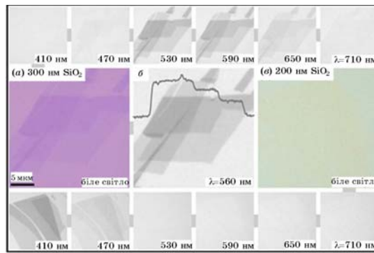
Рис. 3. Зображення «графен на підложжі SiO 2 »: (а) біле світло, товщина діелектрика — 300 нм; (б) зелене світло, товщина діелектрика — 300 нм; (в) біле світло, товщина діелектрика — 200 нм [35].
