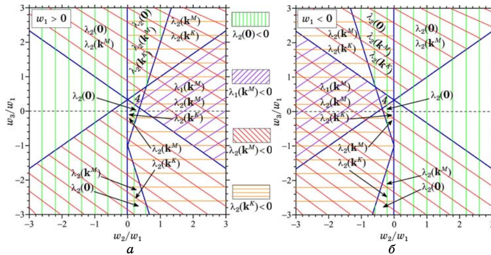
Рис. 22. Ділянки значень параметрів міжатомових взаємодій w_2/w_1 і w_3/w_1 , що «забезпечують» негативність енергетичних параметрів \lambda_2(\mathbf{0}) , \lambda_1(\mathbf{k}^M) , \lambda_2(\mathbf{k}^M) і \lambda_2(\mathbf{k}^K) , а тому й позитивність температур втрати стійкості неупорядкованого стану щодо перетворення його у відповідний впорядкований T_s = -k_B^{-1}c(1-c)\min\lambda_\omega(\mathbf{k}) (4 — ділянка, де негативні всі чотири параметри).
