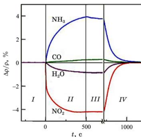
Рис. 15. Зміна провідності (у відсотках) з часом в умовах графенової взаємодії з молекулами \text{NH}_3 , \text{CO} , \text{H}_2\text{O} і \text{NO}_2 . Ділянка I — зразок, розташований у вакуумі, II — зразок в атмосфері гелію чи азоту, III — припинення адсорбції, IV — відпалювання за температури 150^\circ\text{C} [67].
