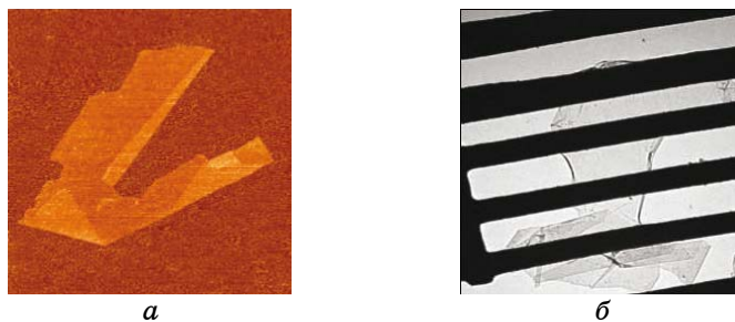
Рис. 7. Графенове зображення (а), одержане за допомогою АСМ, де найтемніша ділянка — \text{SiO}_2 -підложжя, «помаранчеві» ділянки (темніші в черно-білих кольорах) — графен товщиною 0,6 нм, а «жовтогарячі» (світліші в черно-білих кольорах) — графен товщиною 1,2 нм. Підвішений на металевому каркасі графенів шар (б) [50].
