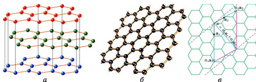
Рис. 1. Графітова (а) й графенова структури (б) та схема «створення» односвітної нанорурки (n_1, n_2) (в) розрізуванням графенової пласкої сітки за напрямками штрихових ліній і згортанням її вздовж напрямку вектора \mathbf{r} [6].
