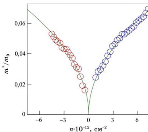
Рис. 10. Залежність циклотронної маси, нормованої на масу спокою вільного електрона m_0 , від концентрації електронів («позитивна» концентрація) і дірок («негативна» концентрація). Кружечки відповідають експериментальним даним, а суцільні лінії — теоретична апроксимація [28].
