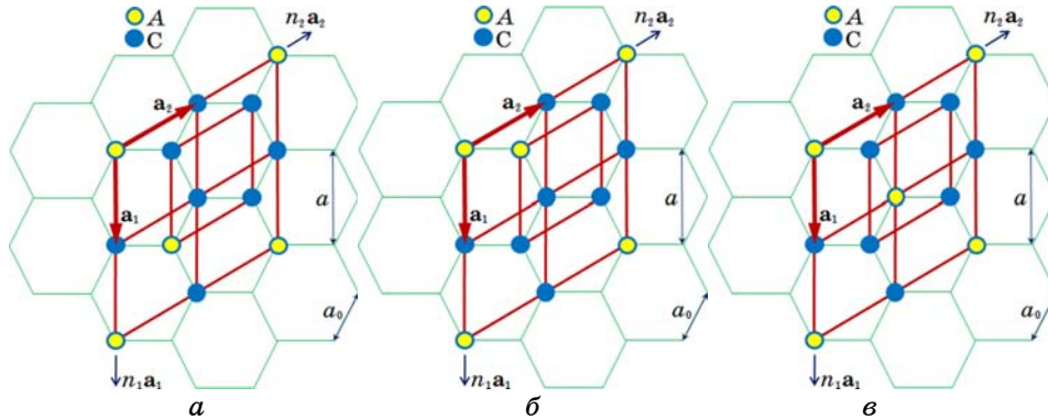
Рис. 19. Примітивні елементарні комірки надструктур зі стехіометрією 1/4 (описуються одним ( a ), двома ( b ) або трьома ( v ) параметрами порядку).
