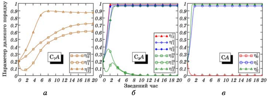
Рис. 29. Часова залежність параметрів далекого порядку систем типу легованих графенових за певних значень температури T^* = k_B T/|\lambda_2(\mathbf{k}^M)| = 0,1 і параметрів взаємодій атомів: \lambda_1(\mathbf{k}^M)/\lambda_2(\mathbf{k}^M) = 5/6 , \lambda_2(\mathbf{0})/\lambda_2(\mathbf{k}^M) = -5/8 ( \lambda_2(\mathbf{k}^M) < 0 ).
