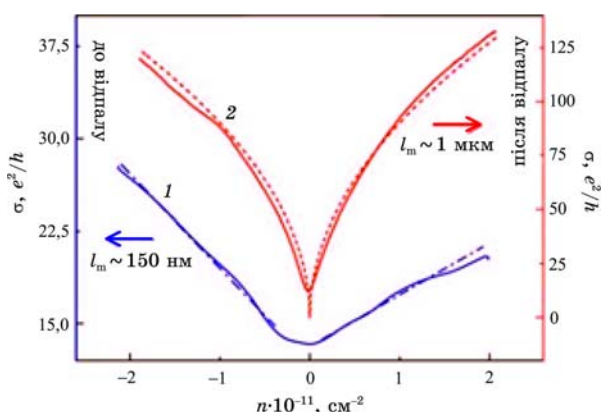
Рис. 12. Графенова провідність до (1) та після (2) відпалу в залежності від концентрації носіїв заряду [63].
