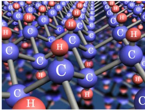
Рис. 16. Кристал графану [105].
