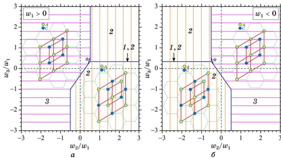
Рис. 24. Те ж саме, що й на рис. 23, але для надструктур типу СА, що описуються одним параметром далекого порядку та мають різні конфігураційні внутрішні енергії, які, крім \lambda_1(\mathbf{0}) , визначаються лише одним параметром міжатомових взаємодій: \lambda_1(\mathbf{k}^M) (1), \lambda_2(\mathbf{k}^M) (2) або \lambda_2(\mathbf{0}) (3). Зірочка «*» позначає діляночку, якій відповідає надструктура (3), що визначається параметром \lambda_2(\mathbf{0}) і була б енергетично найвигіднішою, проте, на ній \lambda_2(\mathbf{0}) > 0 .
