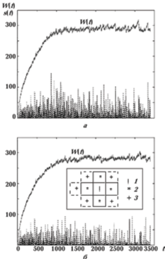
Рис. 3. Изменение во времени общей энергии в решетке и размера лавин в случае с ДД: L = 12 , i_* = 4 , j_* = 10 ( a - z^* = 600 ; b - z^* = 250 ). На врезке: рост кластера клеток ДД (1 — ячейка поступления энергии; 2 — клетки кластера на момент времени t = 1455 ; 3 — новые клетки кластера на момент времени t = 3158 ).
