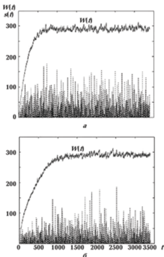
Рис. 2. Изменение во времени общей энергии в решетке W(t) и размера лавин s(t) в случае без ДД: L = 12 , а — i_* = 7 , j_* = 4 ; б — i_* = 4 , j_* = 10 .
