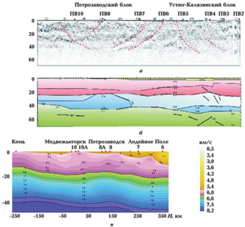
Рис. 7. Сейсмические разрезы по участку геотранверса 1-ЕВ, полученные методами ОГТ (а), ГСЗ (б), и томографический разрез (в). На рис. а красными штриховыми линиями отмечены глубинные нарушения и границы блоков коры; на рис. б — изолинии скорости (км/с), утолщенные линии — отражающие площадки; ПВ — пункты взрыва; на рис. в — изолинии скорости в км/с.
