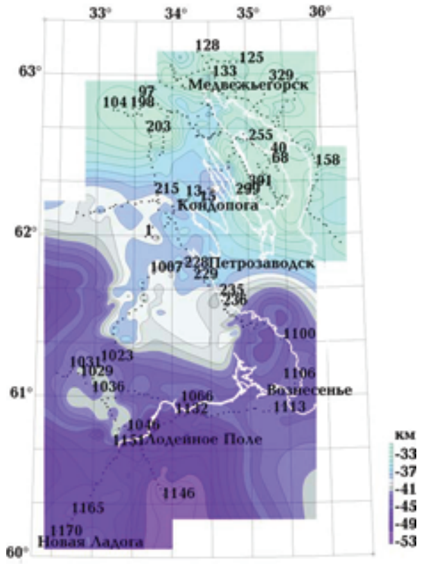
Рис. 9. Мощность земной коры по границе М 1 . Составили Э.В. Исанина, С.И. Южанинова.
