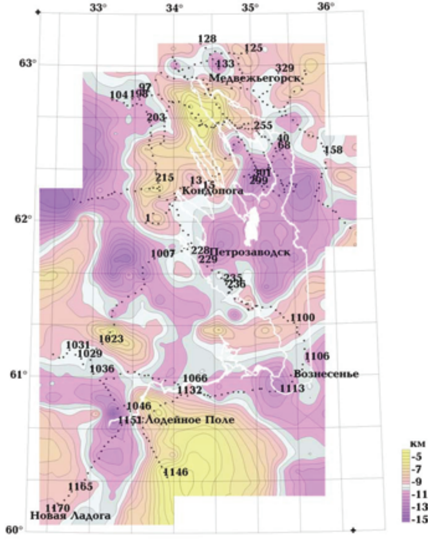
Рис. 10. Мощность коромантийного переходного слоя. Составили Э.В. Исанина, С.И. Южанинова.
