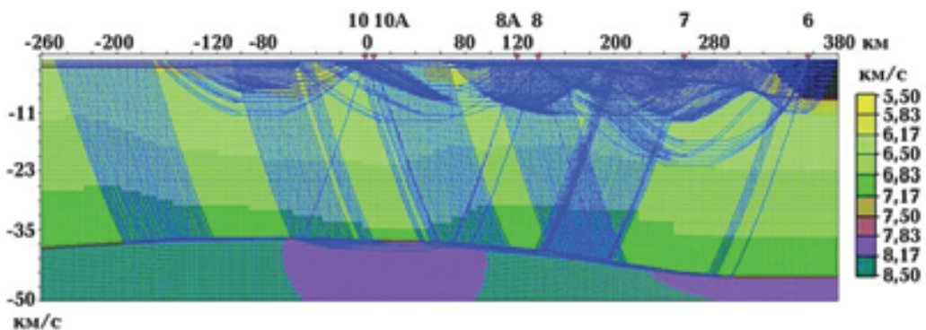
Рис. 6. Результаты сейсотомографического моделирования по участку геотраверса 1-ЕВ, скоростная модель и траектории сейсмических лучей. Составили Э.В. Исанина, Н.А. Крупнова (2010).
