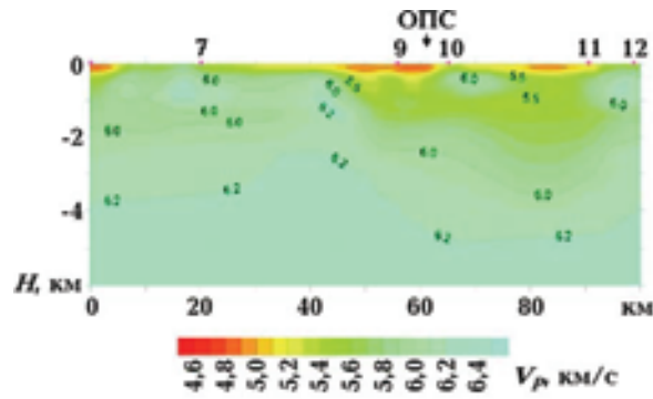
Рис. 4. Результаты сейсотомографического моделирования по профилю Сязозеро — Повенецкий залив. Составили Э.В. Исанина, Н.А. Крупнова, Н.В. Шаров (2009).
