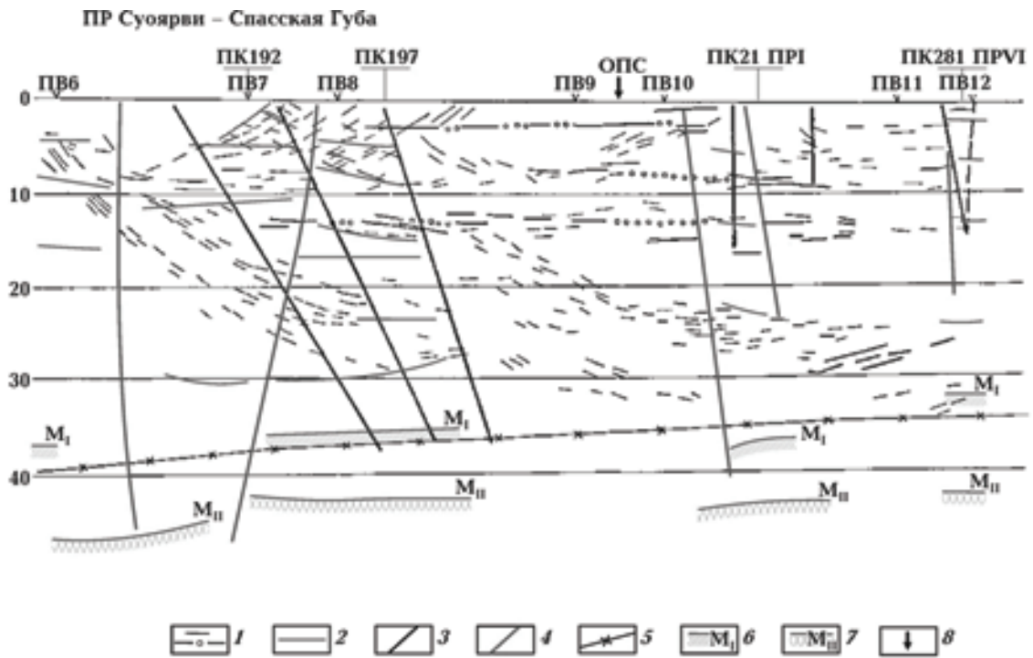
Рис. 3. Сопоставление глубинных разрезов по профилю МОВ, ГСЗ Сямозеро — Повенецкий залив (ЗГТ) и участкам профилей МОВЗ Суоярви — Спасская Губа, I, VI (ГП "Невскгеология"): 1 — границы по данным ГСЗ; 2 — границы по данным МОВЗ; 3 — зоны нарушений по данным ГСЗ; 4 — зоны нарушений по данным МОВЗ; 5 — положение границы М по данным гравиразведки; 6 — положение границы M_I по данным МОВЗ; 7 — положение границы M_{II} по данным МОВЗ; 8 — проекция Онежской параметрической скважины на профиль.
