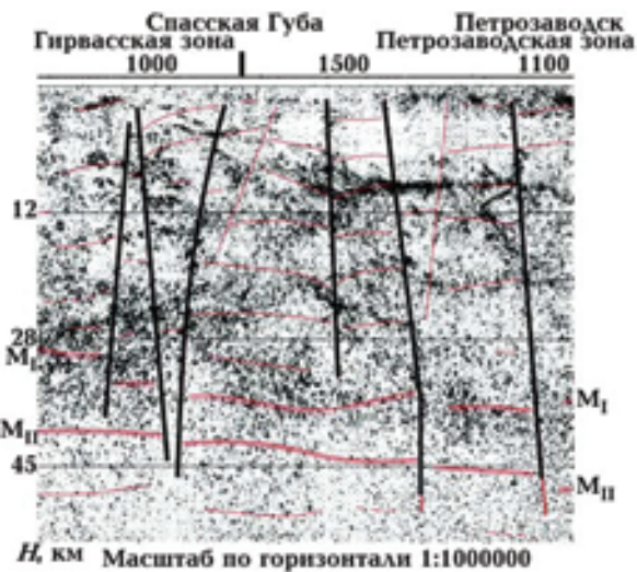
Рис. 8. Совмещенный глубинный разрез ОГТ (ФГУ УГГП “Спецгеофизика”) и МОВЗ (ГП “Невскгеология”) по участку геотранверса 1-ЕВ.
