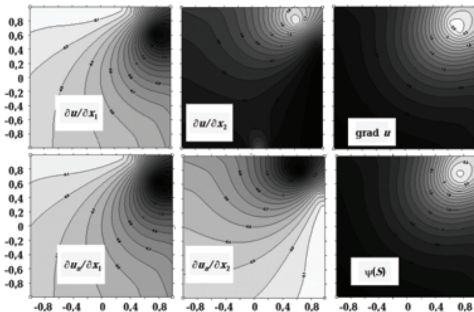
Рис. 3. Решение внутренней граничной задачи (4) для единичного круга.
