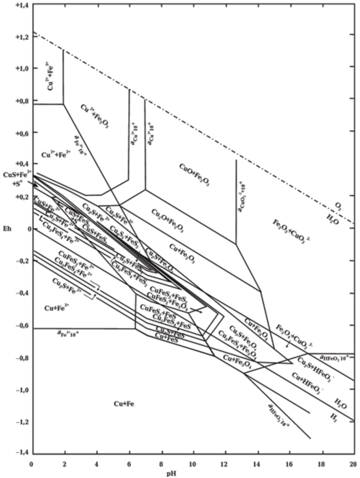
Рис. 1. Система Cu — Fe — S — O — H (медь — железо — вода — сера) при 25 °С и 1 атм общего давления. Сумма растворенной серы 10 -4 моль/л [Гаррелс, Крайт, 1968].
