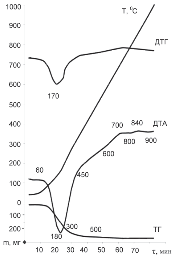
Рис. 1. Результаты термогравиметрического /дифференциального термического анализа осадка гидроксидов циркония, иттрия и европия
