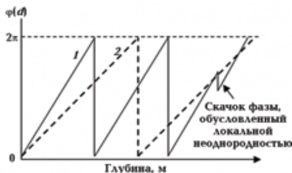
Рис.4. Фазочастотный спектр сигнала, прошедшего либо однородную среду (1), либо среду, в которой находится неоднородность (2).
