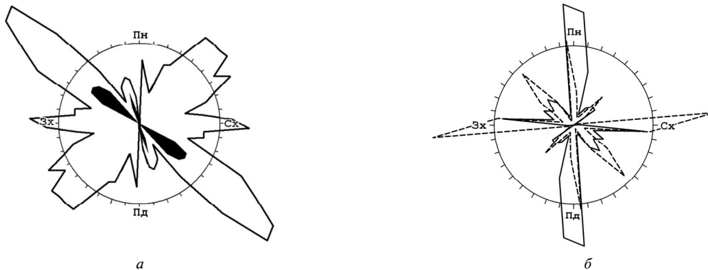
Рис. 5. Порівняння діаграм за суміщенням: a – на прикладі діаграм простягання розломів і дайок Вовчанського виступу Приазовського блока Українського щита; б – на прикладі діаграм простягання розломів Західноінгулецької зони щита, побудовані на основі карт різних авторів
