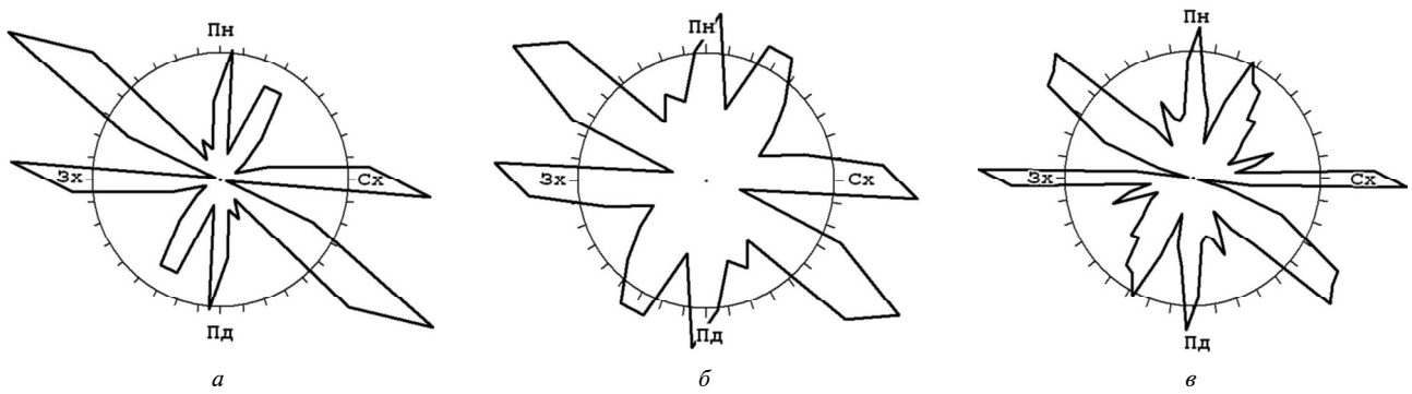
Рис. 4. Підбір параметрів діаграми на прикладі діаграми простягання розломів Вовчанського виступу Приазовського блока Українського щита: a – шкала лінійна, інтервал об’єднання даних 10°; б – шкала корінь квадратний, інтервал об’єднання даних 10°; в – шкала корінь квадратний, інтервал об’єднання даних 5°
