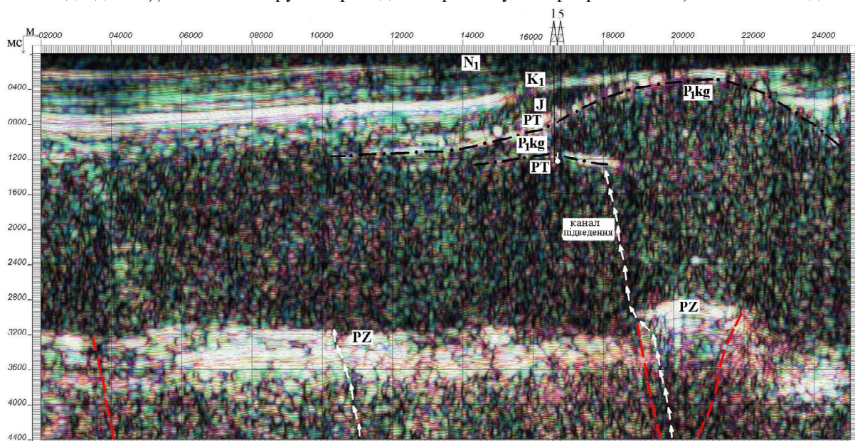
Рис. 3. Сейсмолітологічний розріз
