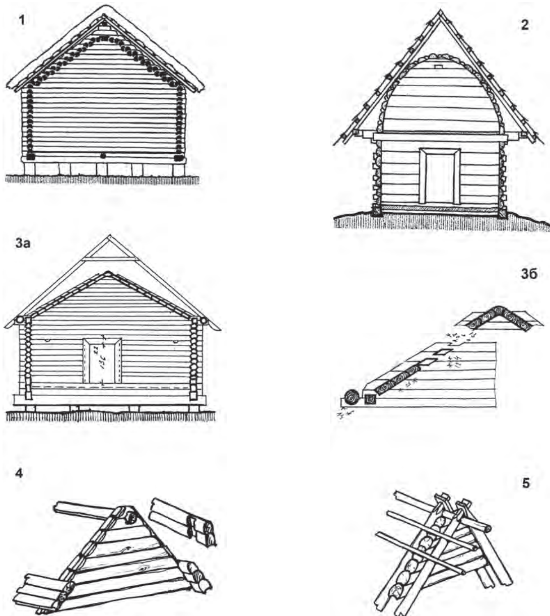
Конструктивні різновиди суцільного накоту: 1 — Кліть із с. Чудина за З. Дмоховським); 2 — «Сипанець» (комора) зі с. Лемківщини (за М. Мушинкою); 3а, 3б — комора зі с. Левковичів Овруцького р-ну Житомирської обл.; 4 — «Амбар» з Молодечинського р-ну Білорусії (за В. Трацевським); 5 — Причілок із колод, затиснутих між двома парами крокв, с. Яловичі Ів'євського р-ну, Білорусія (за В. Трацевським)
