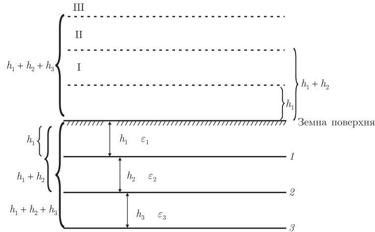
Рис. 1. Модель (фрагмент) земної кори: h_1-h_3 — товщина пластів осадових порід; \varepsilon_1 - \varepsilon_3 — їх діелектрична проникність; 1, 2, 3 — межі пластів; I, II, III — пучність стоячих хвиль
