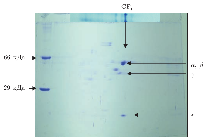
Рис. 3. Електрофореграма пептидного складу чинника спряження тилакоїдних мембран (електрофорез у другому напрямку (система Леммлі)). Субодиниці CF_1 — \alpha (60 кДа), \beta (56 кДа), \gamma (39 кДа), \delta (20,5 кДа), \epsilon (14,7 кДа)
