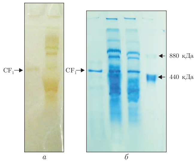
Рис. 2. АТФазна активність білкових зон очищеного чинника спряження після нативного ПААГ електрофорезу: a — АТФазна активність; b — ПААГ, оброблений барвником Кумасі G-250
