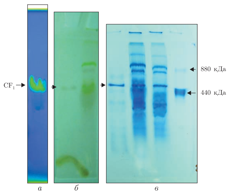
Рис. 4. Карбоангідразна активність білкових зон очищеного чинника спряження після нативного ПААГ електрофорезу: a — ПААГ, забарвлений бромтимоловим синім; б — ПААГ, що інкубували за наявності 2 мМ CoSO_4 ; в — ПААГ, оброблений барвником Кумасі G-250 (880 кДа, 440 кДа — білки-маркери (димер та мономер феретину))
