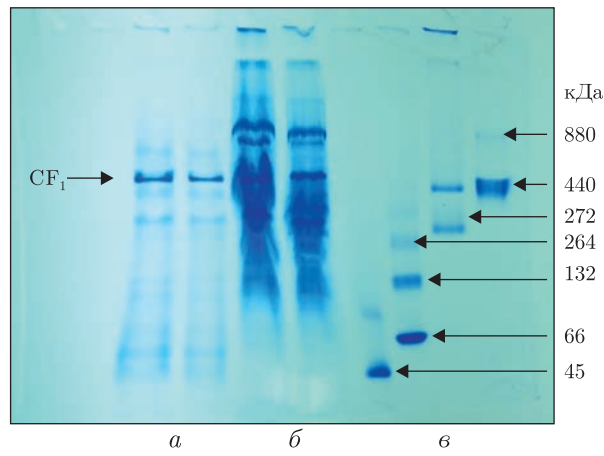
Рис. 1. Електрофореграма нативного білка (безбарвний нативний електрофорез зі зміщенням заряду): a — очищений чинник спряження CF_1 ; b — дигітоніновий солюбілізат тилакоїдів; c — білки-маркери
